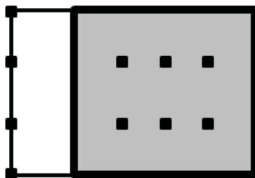
ภาพที่ 3.174 : แบบแปลนพระวิหารแบบที่ 4 รูปแบบที่มีโถงทางเข้าด้านหน้าและด้านหลัง อัตราส่วนส่วนโถงด้านหน้าต่อพื้นที่ภายใน เท่ากับ 1 ต่อ 4 ส่วน
