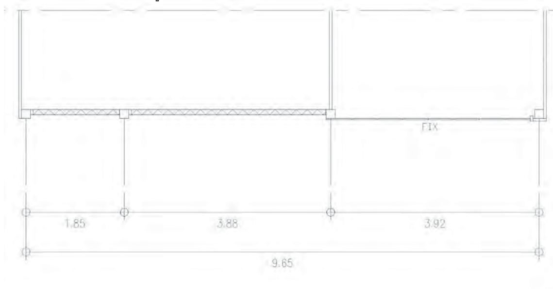
ภาพที่ 3.143 : แปลนอาคาร กลุ่มอาคาร J ร้านญาติเฒ่า
