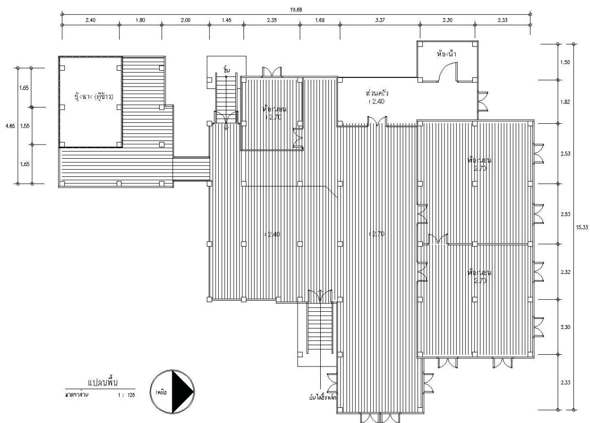
ภาพที่ 3.6: แสดงแปลนบ้าน นางต๋อมแก้ว สุวัง
