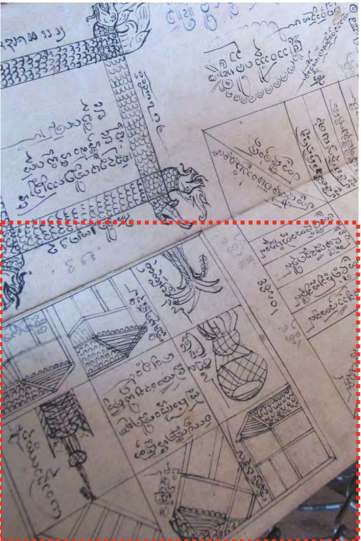
ภาพที่ 3.80 : รูปตารางพิบสา สำหรับกำหนดจำนวนเสาบ้าน
