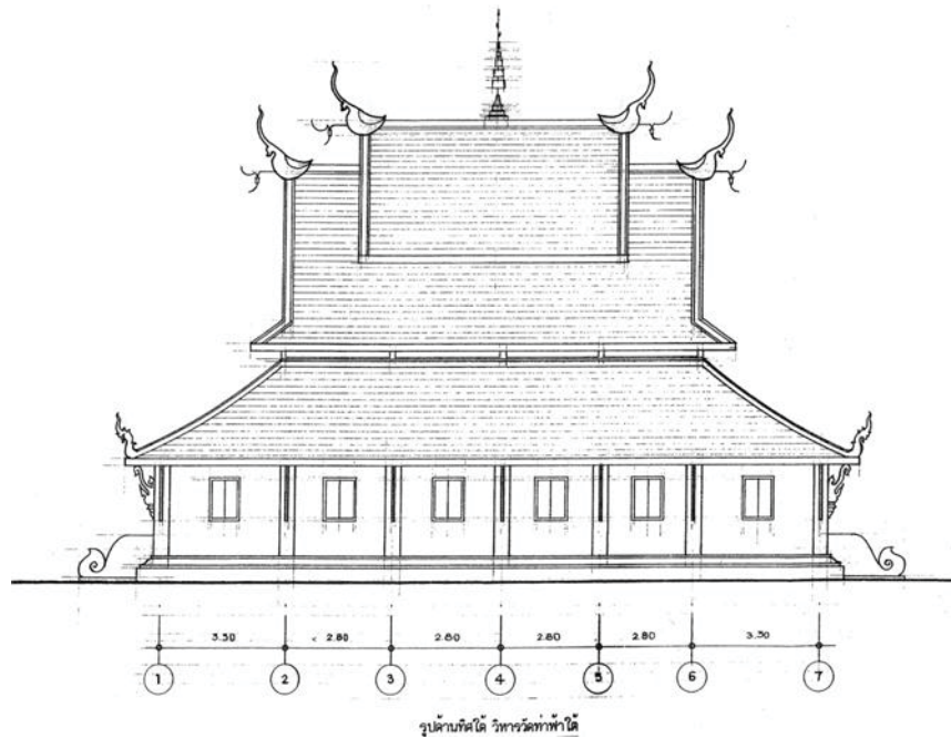
ภาพที่ 3.17: รูปด้านทิศตะวันออก วิหารวัดท่าฟ้าใต้ บ้านฟ้าสีทอง ต.สระ อ.เชียงม่วน จ.พะเยา
