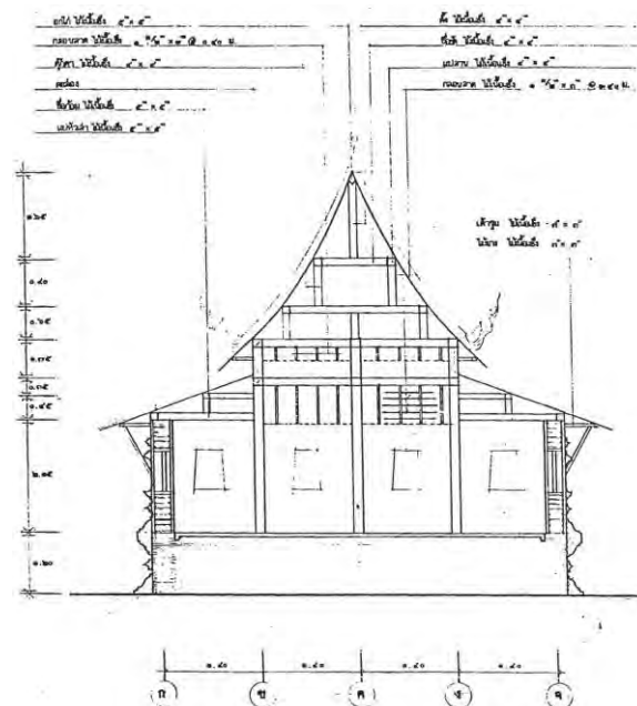
ภาพที่ 3.35:แสดงรูปตัดด้านสกัด หอไตรวัดพระหลวง บ้านพระหลวง ต.พระหลวง อ.สูงเม่น จ.แพร่ ที่มา : ห้างหุ้นส่วนจำกัด เฌอ กรีน, รายงานการขุดค้นศึกษาทางโบราณคดีและการบูรณะ
