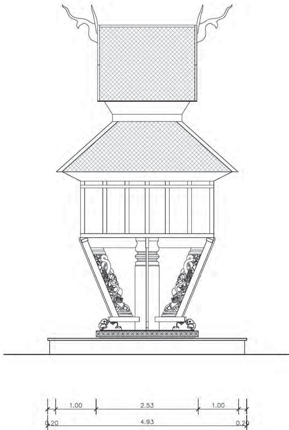
ภาพที่ 3.29 :แสดงแปลนรูปด้านข้าง หอไตรวัดศรีไค้ ต.ศรี อ.เชียงของ จังหวัดเชียงราย ที่มา : โดยอรทัย มหาวรรณและอัมเรศ เทพมาการังวัดตัวอาคารวันที่ 7 พฤศจิกายน 2555
