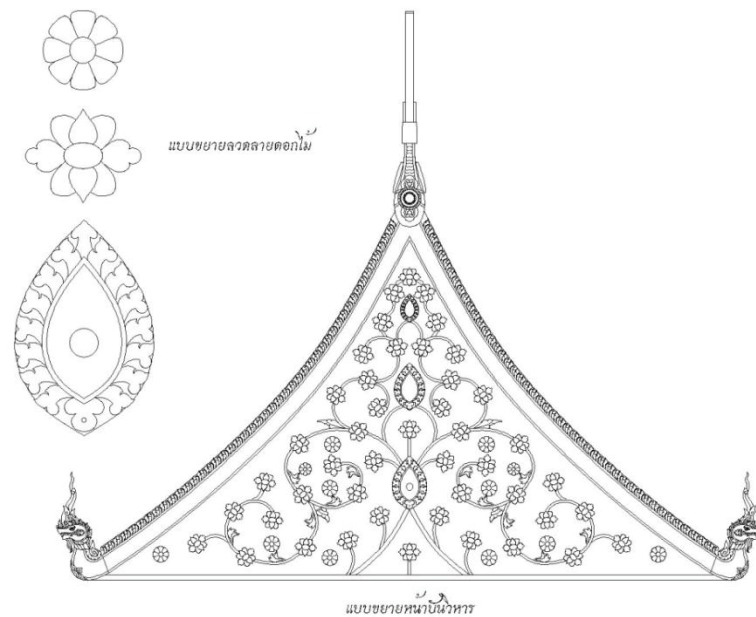
ภาพที่ 3.44 : แสดงแบบขยายหน้าบันและลวดลายบริเวณหน้าบันวิหารวัดท่าฟ้าใต้ ที่มา : โดยอรรถัย มหาวรรณ, จากการลงพื้นที่สำรวจเมื่อวันที่ 27 ตุลาคม พ.ศ.2555
