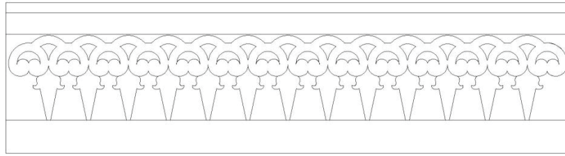
ภาพที่ 3.48 : แสดงแบบขยายลดทอนบริเวณเชิงชายหลังคาวิหารวัดท่าฟ้าใต้ ที่มา : โดย ורתัย มหาวรรณ, จากการลงพื้นที่สำรวจเมื่อวันที่ 27 ตุลาคม พ.ศ.2555
