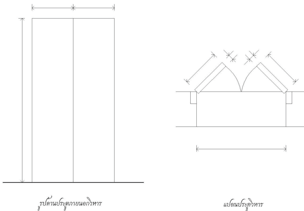
ภาพที่ 3.58 : แสดงแบบขยายประตูวิหารวัดต้นแหลง
