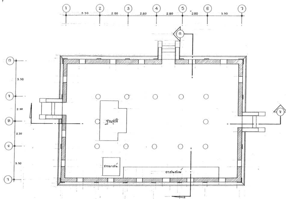
ภาพที่ 3.13 : แสดงแปลนวิหารวัดท่าฟ้าใต้ บ้านฟ้าสีทอง ต.สระ อ.เชียงม่วน จ.พะเยา
