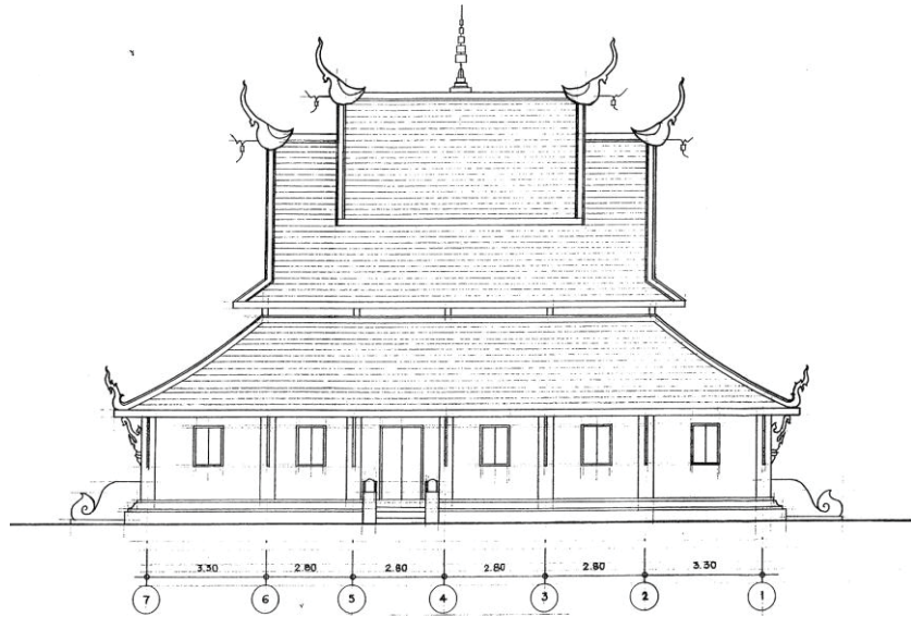
ภาพที่ 3.15: แสดงรูปด้านทิศเหนือ วิหารวัดท่าฟ้าใต้ บ้านฟ้าสีทอง ต.สระ อ.เชียงม่วน จ.พะเยา
