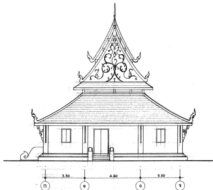
ภาพที่ 3.14 รูปด้านทิศตะวันตก วิหารวัดท่าฟ้าใต้ บ้านฟ้าสีทอง ต.สระ อ.เชียงม่วน จ.พะเยา
