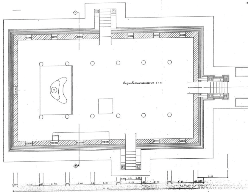
ภาพที่ 3.21 :แสดงแปลนวิหารวัดต้นแหลง บ้านต้นแหลง ต.ชัยวัฒนา อ.ปัว จ.น่าน ที่มา : นายกอบยศ ยิ้มอ่อน, การศึกษาวิหารไตลื้อในวัฒนธรรมล้านนา (จังหวัดพะเยาและจังหวัดน่าน) หน้าที่ 83
