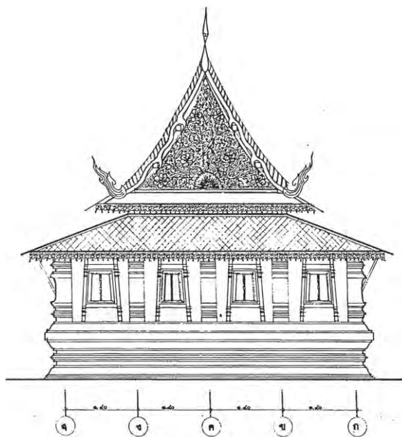
ภาพที่ 3.34:แสดงรูปด้านทิศตะวันออก หอไตรวัดพระหลวง บ้านพระหลวง ต.พระหลวง อ.สูงเม่น จ.แพร่ ที่มา : ห้างหุ้นส่วนจำกัด เฌอ กรีน, รายงานการขุดค้นศึกษาทางโบราณคดีและการบูรณะโบราณสถานวัด พระหลวง หน้าที่ 62
