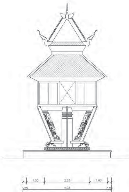
ภาพที่ 3.28:แสดงแปลนรูปด้านหน้า หอไตรวัดศรีไ้ ต.ศรี อ.เชียงของ จังหวัดเชียงราย ที่มา : โดยอรทัย มหารรรณและอัมเรศ เทพมาการังวัดตัวอาคารวันที่ 7 พฤศจิกายน 2555
