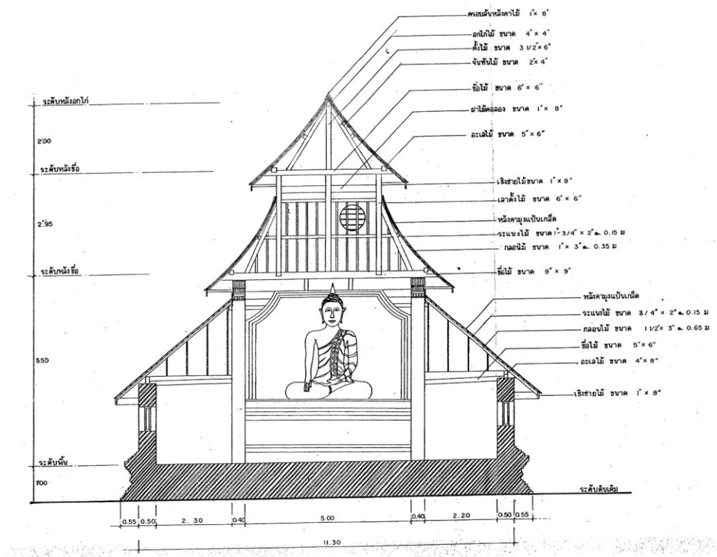
ภาพที่ 3.24 :แสดงรูปตัดด้านสกัด วิหารวัดต้นแหลง บ้านต้นแหลง ต.ชัยวัฒนา อ.ปัว จ.น่าน ที่มา : นายกอบยศ ยิ้มอ่อน, การศึกษาวิหารไดลื้อในวัฒนธรรมล้านนา (จังหวัดพะเยาและจังหวัดน่าน) หน้าที่ 86
