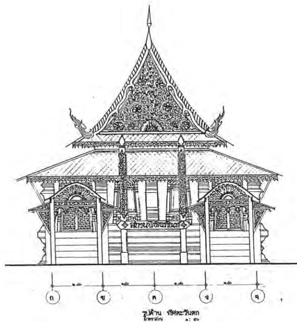
ภาพที่ 3.32:แสดงรูปด้านทิศตะวันตก หอไตรวัดพระหลวง บ้านพระหลวง ต.พระหลวง อ.สูงเม่น จ.แพร่ ที่มา : ห้างหุ้นส่วนจำกัด เฌอ กรีน, รายงานการขุดค้นศึกษาทางโบราณคดีและการบูรณะโบราณสถานวัด พระหลวง หน้าที่ 61
