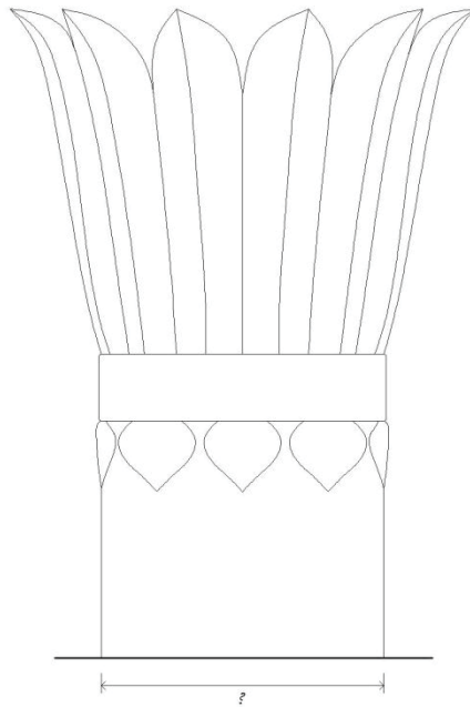
ภาพที่ 3.53 : แสดงแบบขยายลดทอนบริเวณบัวหัวเสาภายในวิหารวัดท่าฟ้าใต้ ที่มา : โดยอรทัย มหารวรรณ, จากการลงพื้นที่สำรวจเมื่อวันที่ 27 ตุลาคม พ.ศ.2555
