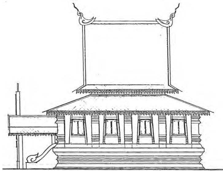
ภาพที่ 3.33 : แสดงรูปด้านทิศใต้ หอไตรวัดพระหลวง บ้านพระหลวง ต.พระหลวง อ.สูงเม่น จ.แพร่ ที่มา : ห้างหุ้นส่วนจำกัด เฌอ กรีน, รายงานการขุดค้นศึกษาทางโบราณคดีและการบูรณะ โบราณสถานวัดพระหลวง หน้าที่ 63
