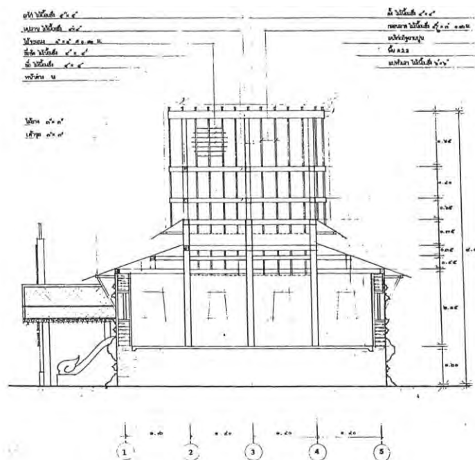
ภาพที่ 3.36:แสดงรูปตัดตามยาว หอไตรวัดพระหลวง บ้านพระหลวง ต.พระหลวง อ.สูงเม่น จ.แพร่ ที่มา : ห้างหุ้นส่วนจำกัด เฌอ กรีน, รายงานการขุดค้นศึกษาทางโบราณคดีและการบูรณะ
