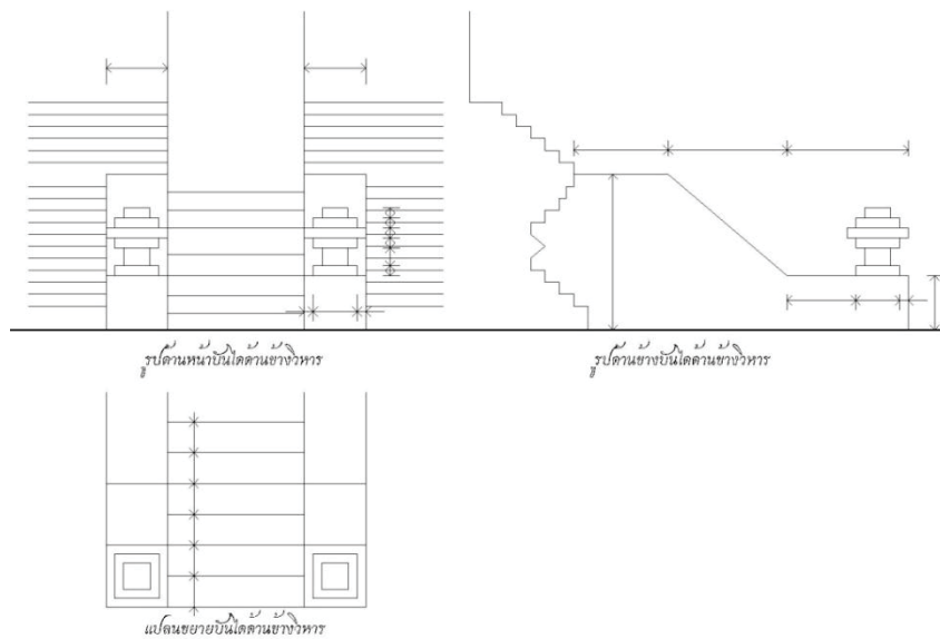
ภาพที่ 3.56 : แสดงแบบขยายบันไดทางเข้าด้านข้างวิหารวัดต้นแหลง
