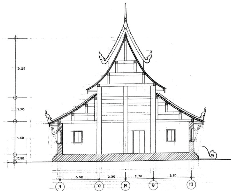
ภาพที่ 3.18: แสดงรูปตัดตามขวาง วิหารวัดท่าฟ้าใต้ บ้านฟ้าสีทอง ต.สระ อ.เชียงม่วน จ.พะเยา
