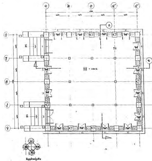
ภาพที่ 3.31:แสดงแปลน หอไตรวัดพระหลวง บ้านพระหลวง ต.พระหลวง อ.สูงเม่น จ.แพร่ ที่มา : ห้างหุ้นส่วนจำกัด เฌอ กรีน, รายงานการขุดค้นศึกษาทางโบราณคดีและการบูรณะ โบราณสถานวัดพระหลวง หน้าที่ 66
