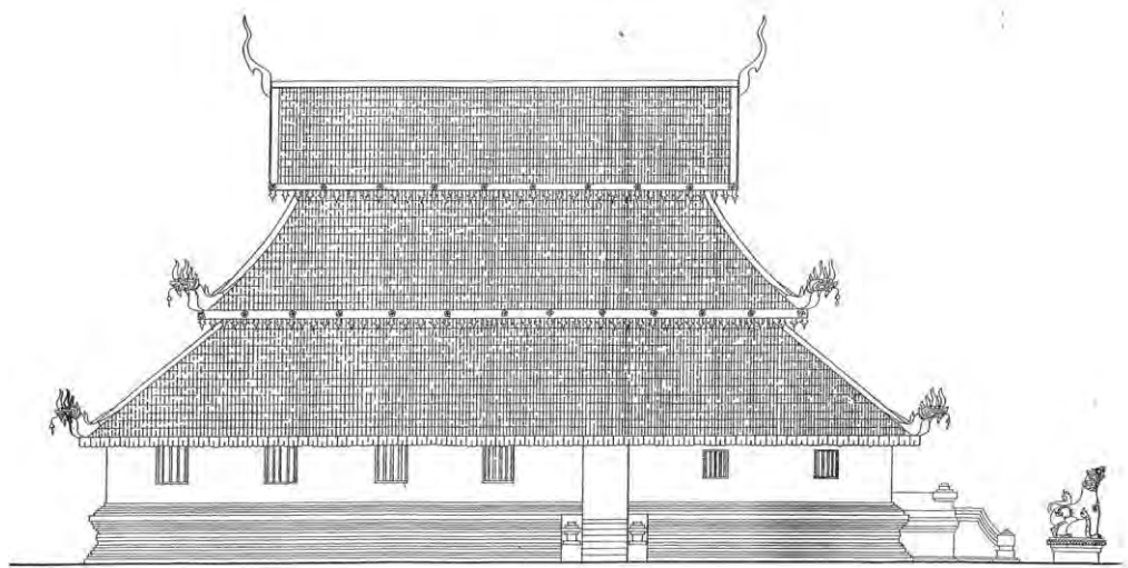
ภาพที่ 3.23 :แสดงรูปด้านทิศใต้ วิหารวัดต้นแหลง บ้านต้นแหลง ต.ชัยวัฒนา อ.ปัว จ.น่าน ที่มา : นายกอบยศ ยิ้มอ่อน, การศึกษาวิหารไดลื้อในวัฒนธรรมล้านนา (จังหวัดพะเยาและจังหวัดน่าน) หน้าที่ 84
