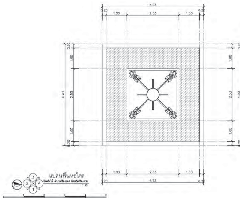
ภาพที่ 3.26 :แสดงแปลนพื้นหอไตรวัดศรีโสดา ต.ศรี อ.เมือง จังหวัดเชียงราย
