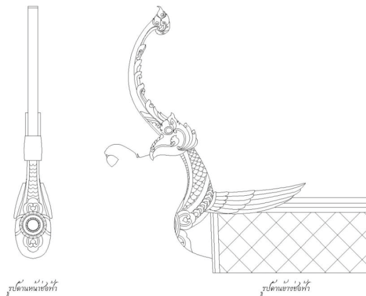
ภาพที่ 3.45 : แสดงแบบขยายหอพักหลังคาวิหารวัดท่าฟ้าใต้ ที่มา : โดยอรรถัย มหาวรรณ, จากการลงพื้นที่สำรวจเมื่อวันที่ 27 ตุลาคม พ.ศ.2555
