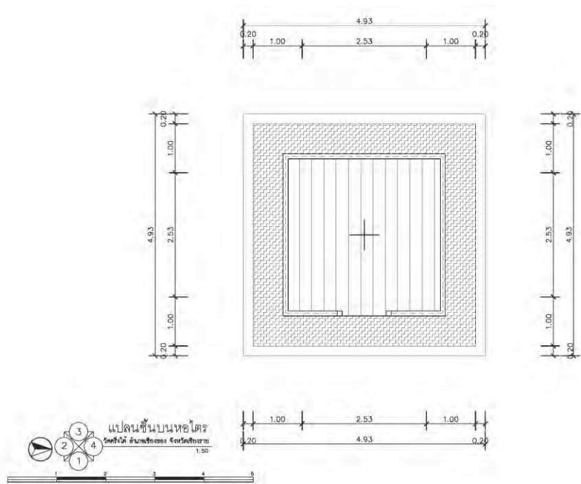
ภาพที่ 3.27:แสดงแปลนชั้นสองหอไตรวัดศรีไ้ ต.ศรี อ.เชียงของ จังหวัดเชียงราย ที่มา : โดยอรทัย มหารรรณและอัมเรศ เทพมาการังวัดตัวอาคารวันที่ 7 พฤศจิกายน 2555
