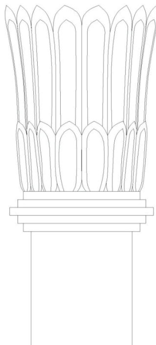
ภาพที่ 3.60 : แสดงแบบขยายลวดลายบริเวณบัวหัวเสาภายในวิหารวัดตันแหง
