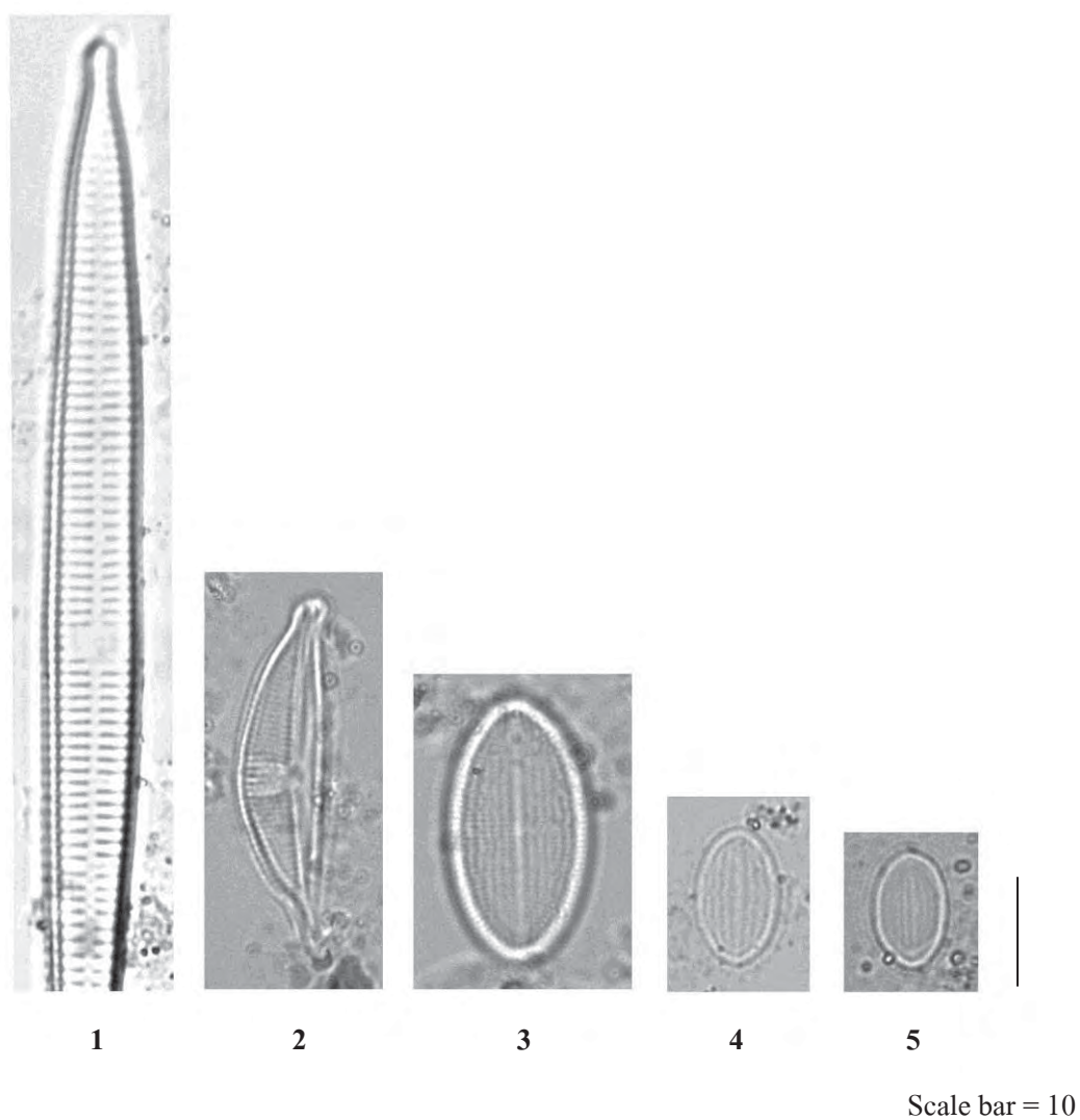
ภาพที่ 4.23 ไดอะตอมพื้นท้องน้ำที่พบในห้วยแม่ลู ตำบลเชียงดาว อำเภอเชียงดาว จังหวัดเชียงใหม่ ของแต่ละจุดเก็บตัวอย่าง ในเดือนกรกฎาคม, พฤศจิกายน และธันวาคม 2555 (1) Synedra ulna var. aequalis (Kützing), (2) Amphora sp. , (3-5) Cocconeis placentula Ehrenberg
