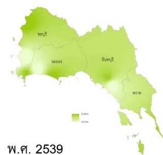
ภาพที่ 4-1 อุณหภูมิเฉลี่ยต่ำสุดรายปี ตั้งแต่ พ.ศ. 2525-2554
