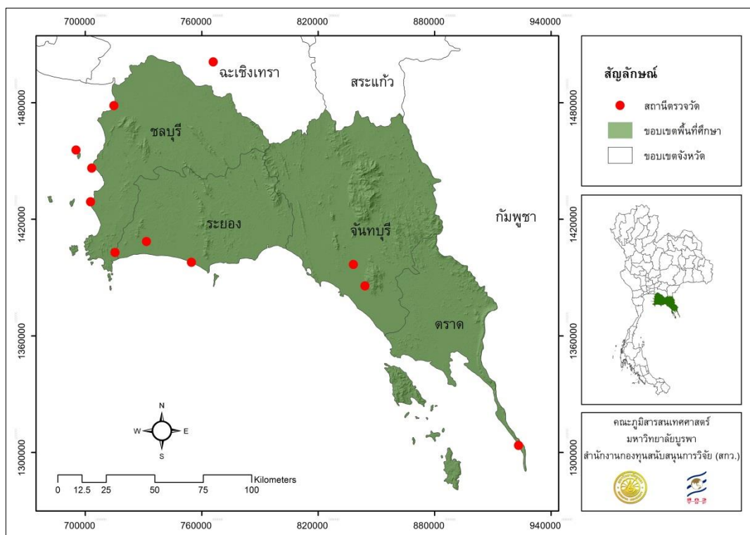
ภาพที่ 3-1 สถานีตรวจวัดอุณหภูมิ ปริมาณน้ำฝน และปริมาณการคายระเหยจากผิวดิน ในจังหวัดชลบุรี ระยอง จันทบุรี และตราด
