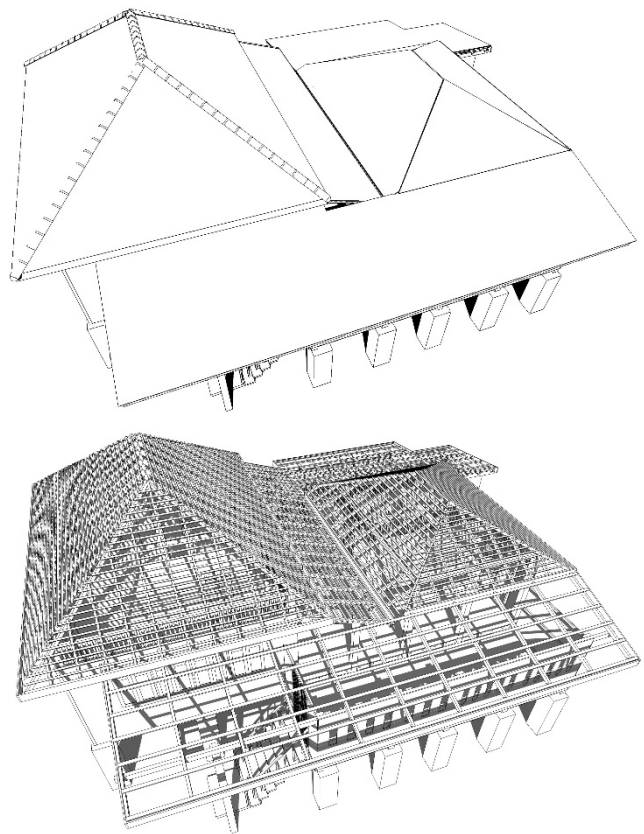
ภาพที่ 4.212 หลังคาทรงปั้นหยาและโครงหลังคา
