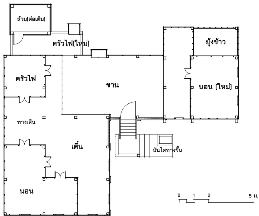
ภาพที่ 4.198 ผังพื้นเรือน
