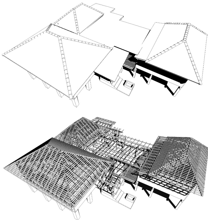
ภาพที่ 4.199 หลังคาบ้านหยาและโครงหลังคา
