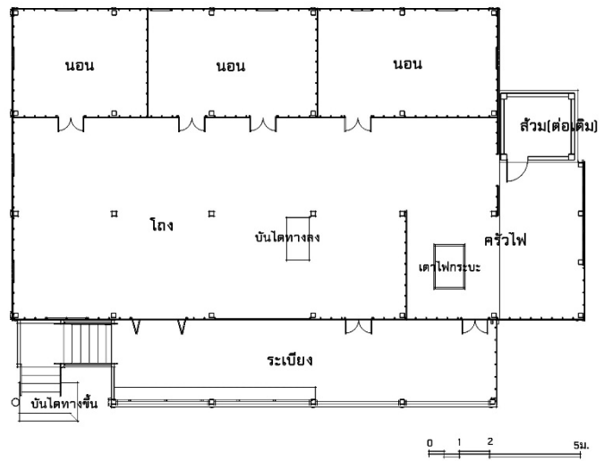
ภาพที่ 4.179 ผังพื้นเรือน
