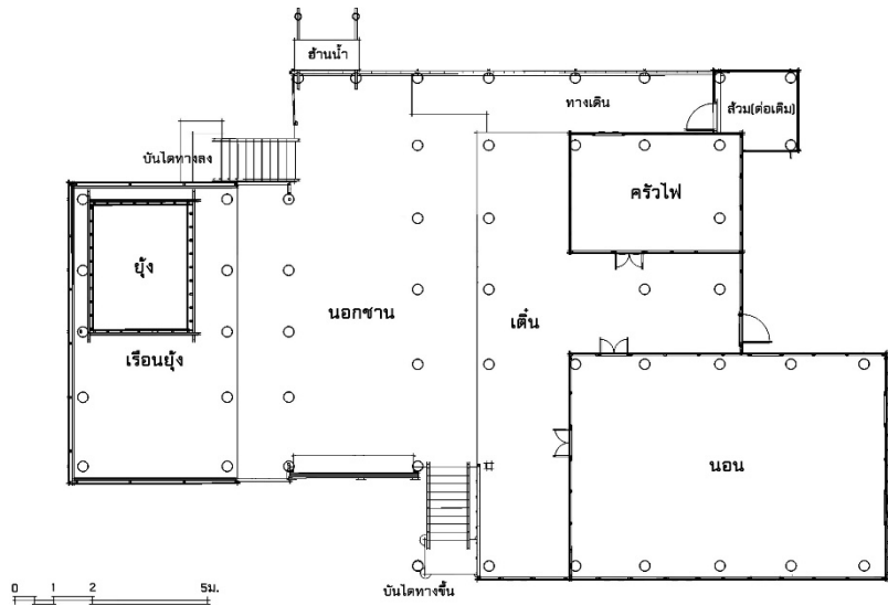
ภาพที่ 4.166 ผังพื้นเรือน
