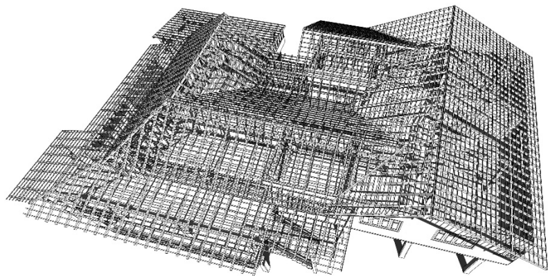
ภาพที่ 4.188 โครงหลังคาเรือน
