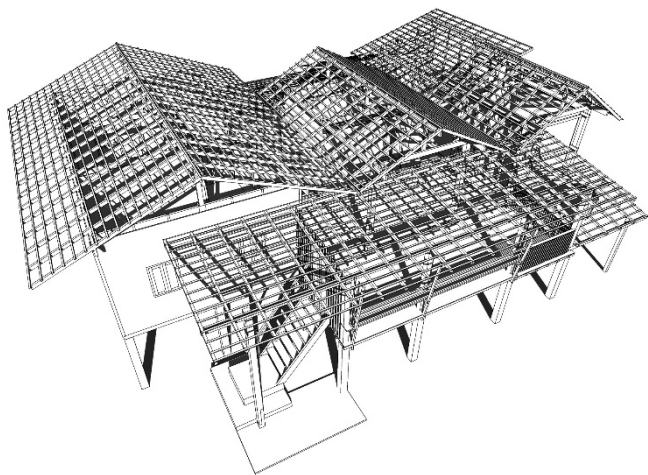
ภาพที่ 4.206 รูปทรงหลังคาและโครงหลังคา
