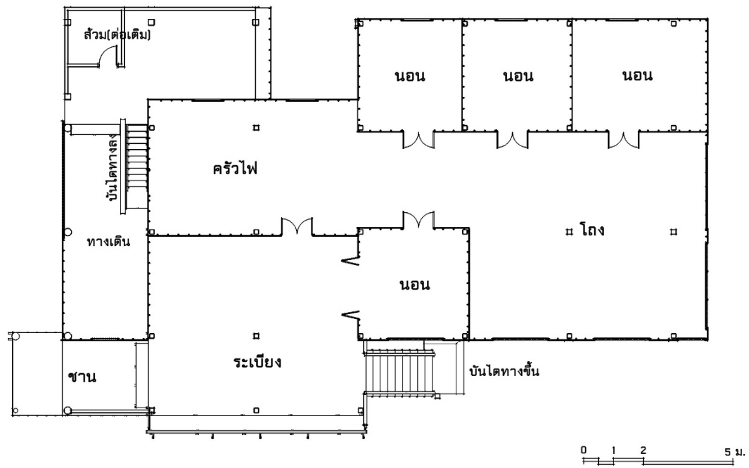
ภาพที่ 4.186 ผังพื้นเรือน
