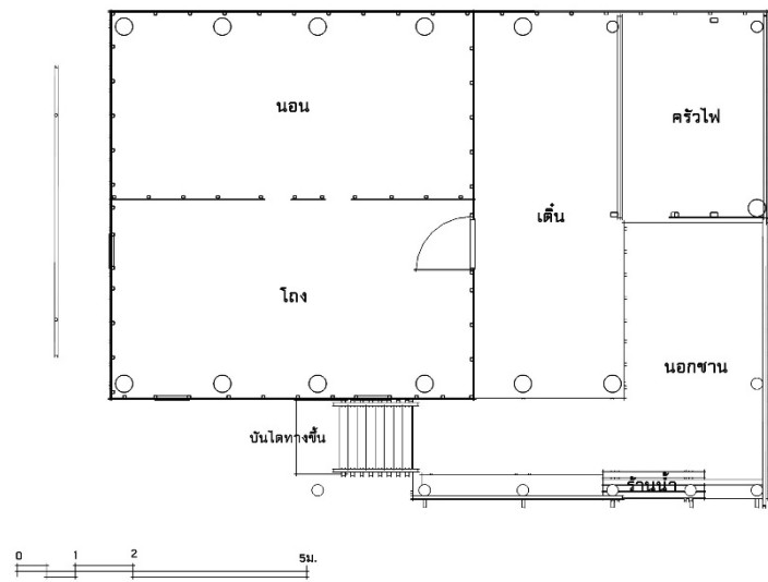
ภาพที่ 4.172 ผังพื้นเรือน
