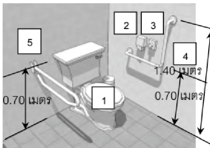
รูปที่ 6.50 หลักการในการออกแบบห้องน้ำเพื่อคนทุกประเภท
