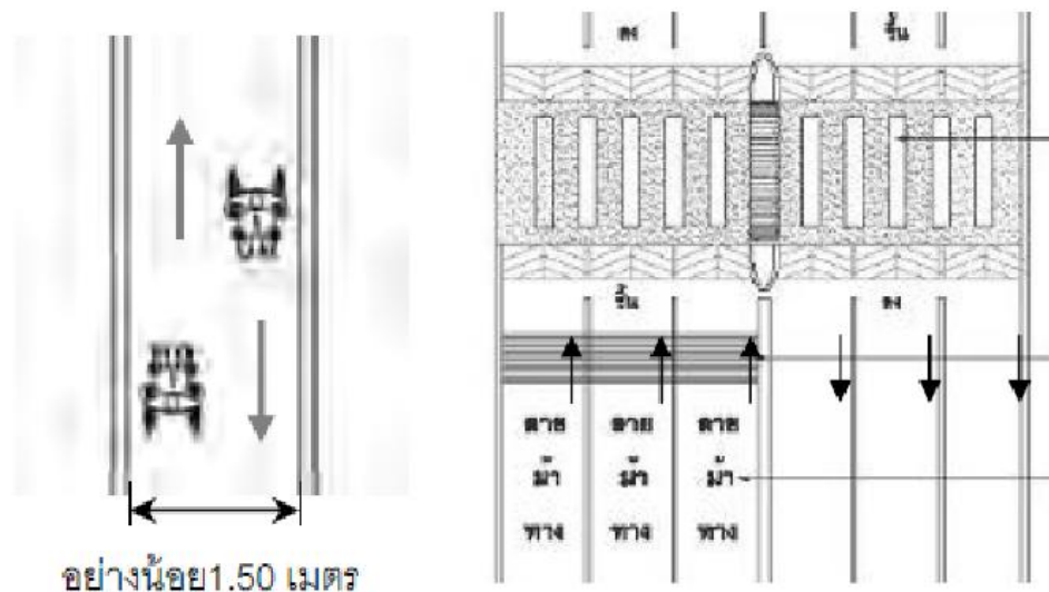
รูปที่ 6.28: หลักการการออกแบบทางเท้าและทางข้าม
