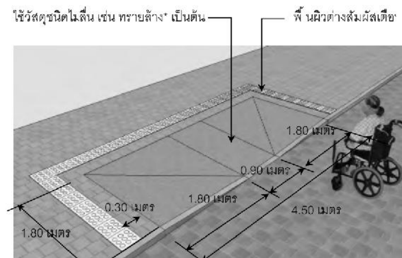
รูปที่ 6.31: หลักการออกแบบทางลาดทางข้ามทางสัญจร
