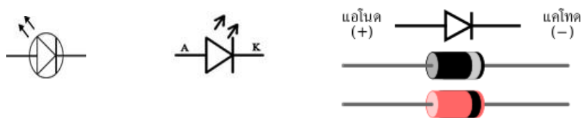
ภาพ 4-1 สัญลักษณ์ของไดโอดเปล่งแสง
