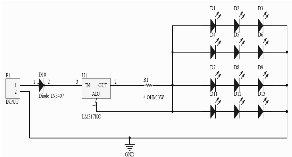
ภาพ 4-2 วงจรโคไฟแอลอีดี
