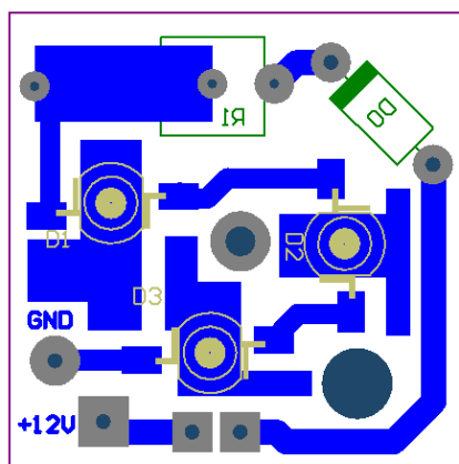
ภาพ 4-5 ลายวงจรพิมพ์โคมไฟแอลอีดีสำหรับใช้ภายในบ้าน
