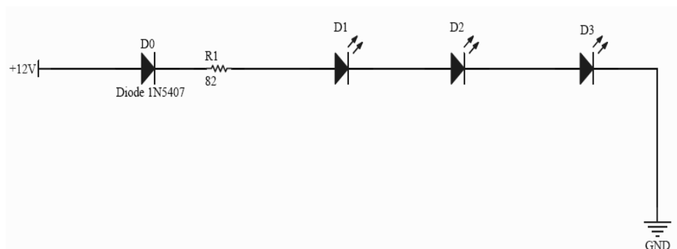
ภาพ 4-4 วงจรโคมไฟแอลอีดีสำหรับใช้ภายในบ้าน
