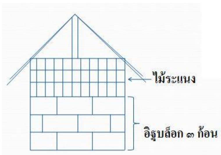
ภาพที่ ๔ - ๑๘ รูปแบบโรงเรือนหมูหลุมแบบคอนโด
