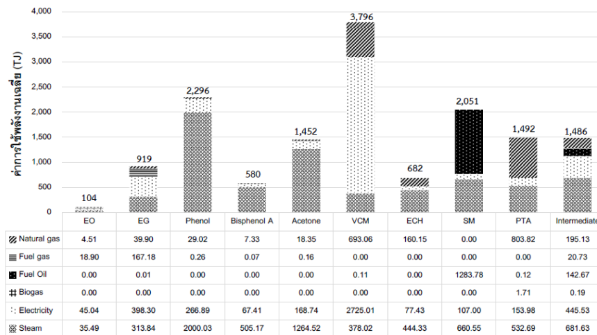
รูปที่ 2-6 ค่าเฉลี่ยการใช้พลังงานโรงงานตัวแทนปิโตรเคมีขั้นกลาง
