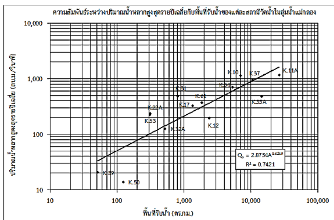
ภาพที่ 2-27 กราฟความสัมพันธ์ระหว่างปริมาณน้ำไหลสูงสุดรายปีเฉลี่ยกับพื้นที่รับน้ำของแต่ละสถานีวัดน้ำในลุ่มน้ำแม่กลอง
