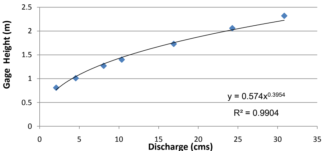
ภาพที่ 4-36 Rating curve ของลำธารห้วยกุยมั่ง บริเวณด้านข้างพูนน้ำร้อนหินดาด
