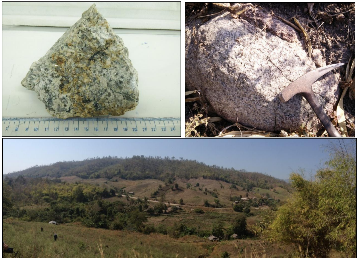
ภาพที่ 4-39 หินแกรนิตผุ (Weathered granite) พบบริเวณภูเขาโค้งมนด้านตะวันตกของพื้นที่ศึกษา (ดอยเกี๊ยะ)
