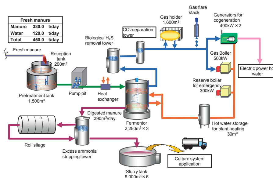
Fig. C3 Recycling new biogas, CO_2 , H_2 , H_2O , NO_x emission
