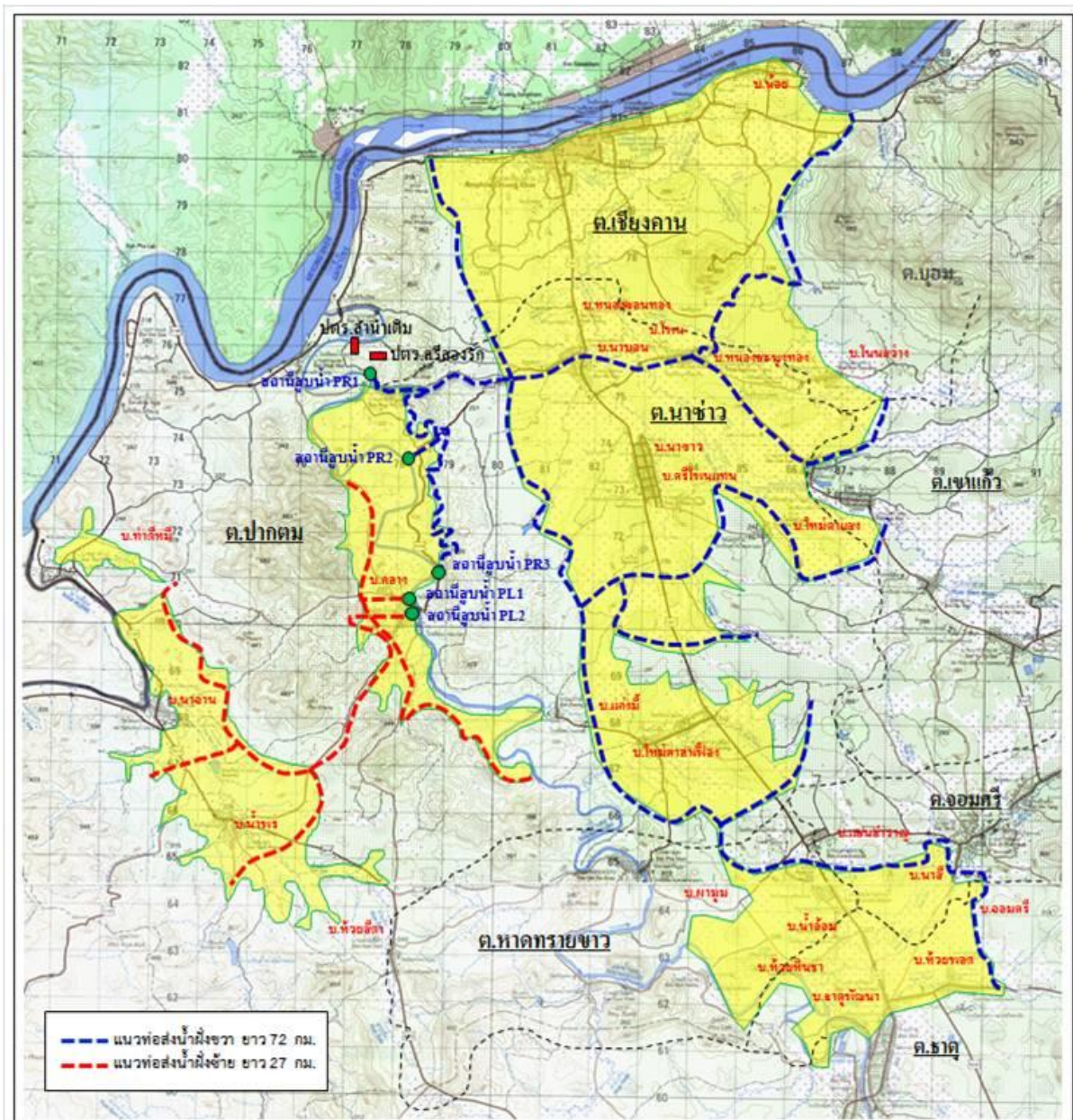
ภาพแสดงระบบท่อส่งน้ำและพื้นที่รับประโยชน์โครงการ
