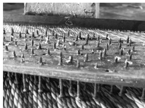
ที่ตรุนสาคุแบบแปรงตะปู
