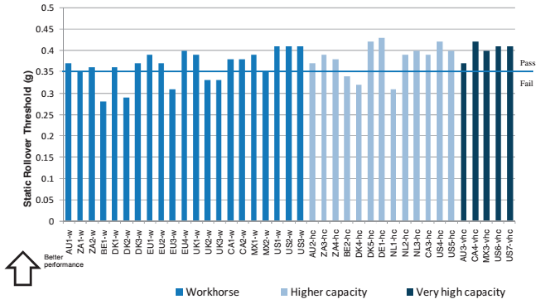
รูปที่ 5.1-4 ผลการวิเคราะห์สมรรถนะรถบรรทุกสำหรับค่า SRT [5]
