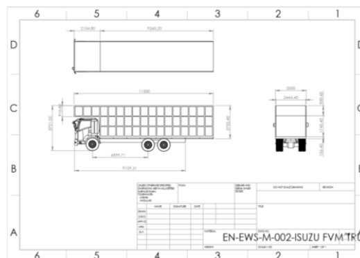
รูปที่ 7.1-7 การปรับปรุงตะกร้ารถบรรทุกสลิบล้อแบบตะแกรง
