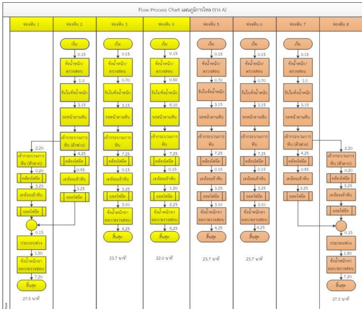
รูปที่ 4.1-41 ขั้นตอนกระบวนการไหลและการเคลื่อนย้ายของวัตถุดิบตั้งแต่ห้องขนถ่ายน้ำหนักรถบรรทุกอ้อย จนสิ้นสุดกระบวนการในร่าง A ที่มา: คณะผู้วิจัย
