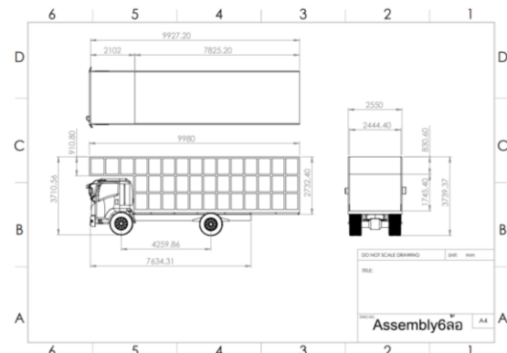
รูปที่ 7.1-9 การออกแบบดัดแปลงตะกร้ารถบรรทุกหกล้อแบบตะแกรง
