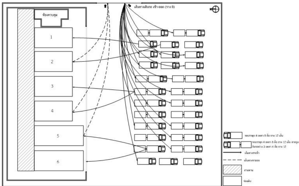
รูปที่ 4.1-40 แผนภาพการไหลและการบริหารจัดการน้ำลานหีบอ้อย ราง B
