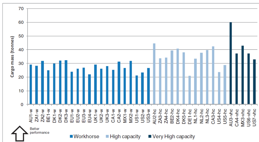
รูปที่ 5.1-1 สมรรถนะการบรรทุกด้านพิกัดน้ำหนัก (cargo mass capacity)
