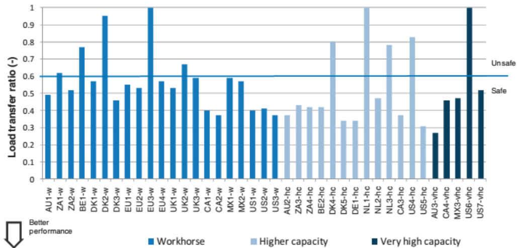
รูปที่ 5.1-8 ผลการวิเคราะห์สมรรถนะรถบรรทุกสำหรับค่า LTR [5]
