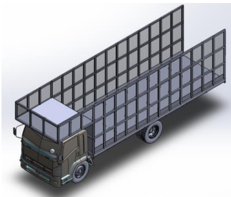
รูปที่ 7.1-9 การออกแบบดัดแปลงตะกร้ารถบรรทุกหกล้อแบบตะแกรง
