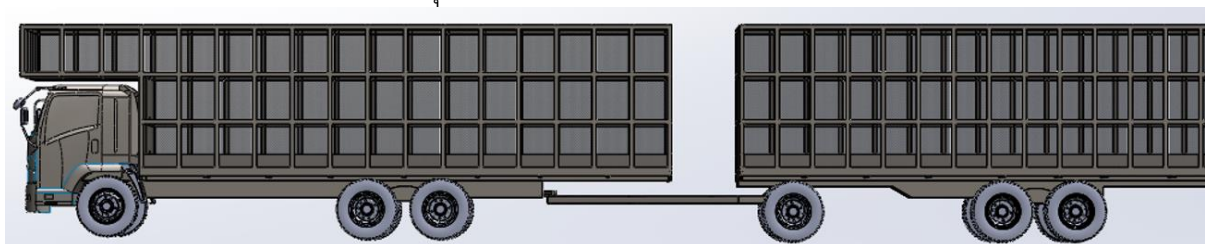
(ค) รถบรรทุกสามเพลา หกล้อ ยางสิบเส้น พร้อมรถลูกฟ่งสามเพลา หกล้อ ยางสิบสองเส้น (3/6/10 + 3/6/12)
