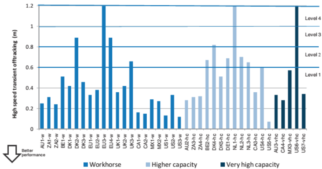
รูปที่ 5.1-7 ผลการวิเคราะห์สมรรถนะรถบรรทุกสำหรับค่า HSTO [5]
