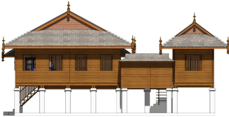
ภาพที่ 49 รูปด้าน B คຸ້ມເຈ້ຍອດເຣືອນ
