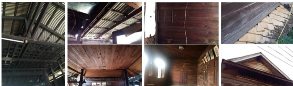
ภาพที่ 37 ภาพแสดงความเสียหายหลังคา บ้านสล่าวงศ์
