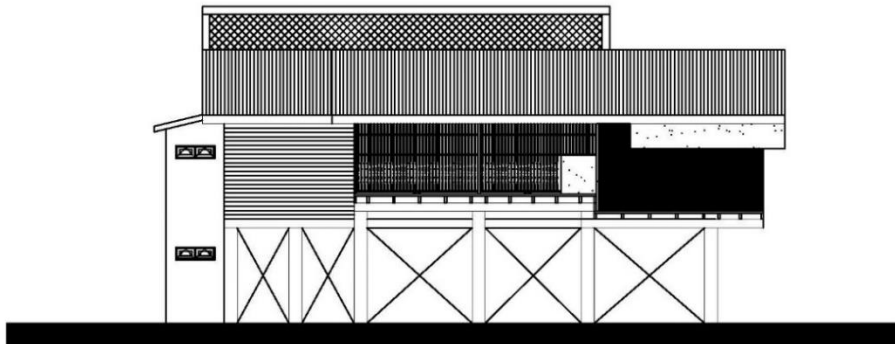
ภาพที่ 72 รูปด้าน B บ้านสว่างค์
