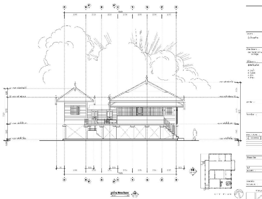
ภาพที่ 65 รูปด้าน B คุ้มเจ้ายอดเรือน
