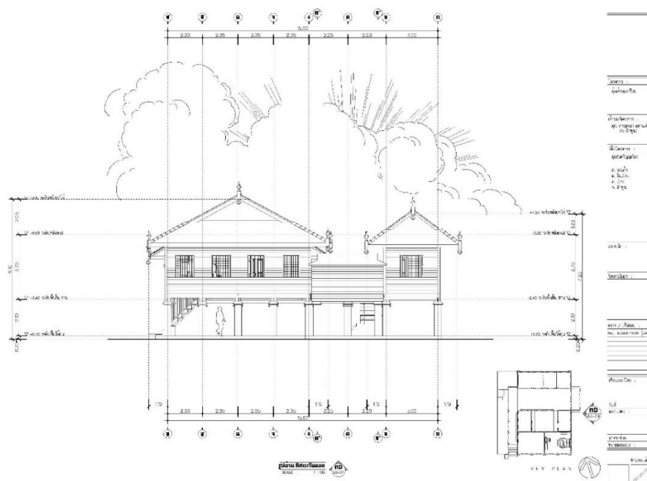
ภาพที่ 67 รูปด้าน D คุ้มเจ้ายอดเรือน
