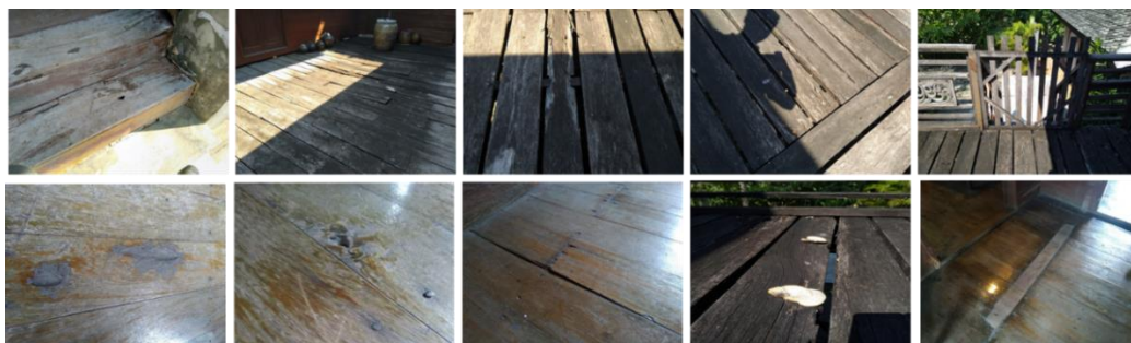
ภาพที่ 30 ภาพแสดงความเสียหายพื้น คຸ້ມເຈ້ຍອຸດເຣືອນ
