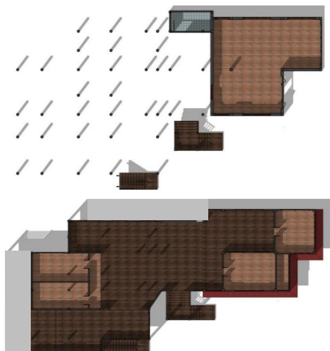
ภาพที่ 44 แปลนพื้นบ้านสล่าวงศ์ในรูปแบบดั้งเดิม
