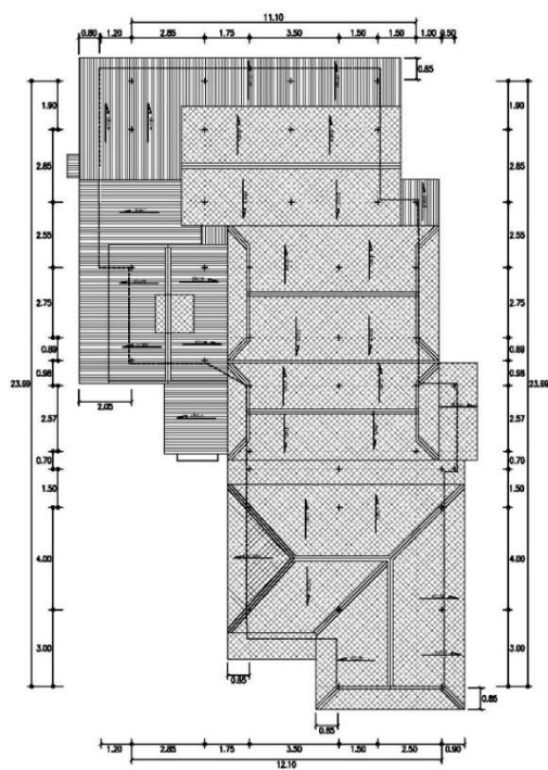
ภาพที่ 70 แพลนหลังคา บ้านสว่างค์
