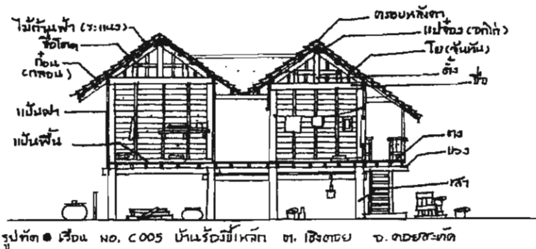
รูป 8.27 รูปตัดของเรือนไทเขินเชียงใหม่ บ้านเลขที่ 33 หมู่ 7 บ้านร่องขี้เหล็ก ตำบลเจริญชัย อำเภอดอยสะเก็ด จังหวัดเชียงใหม่ ของนายยืน สายกา
