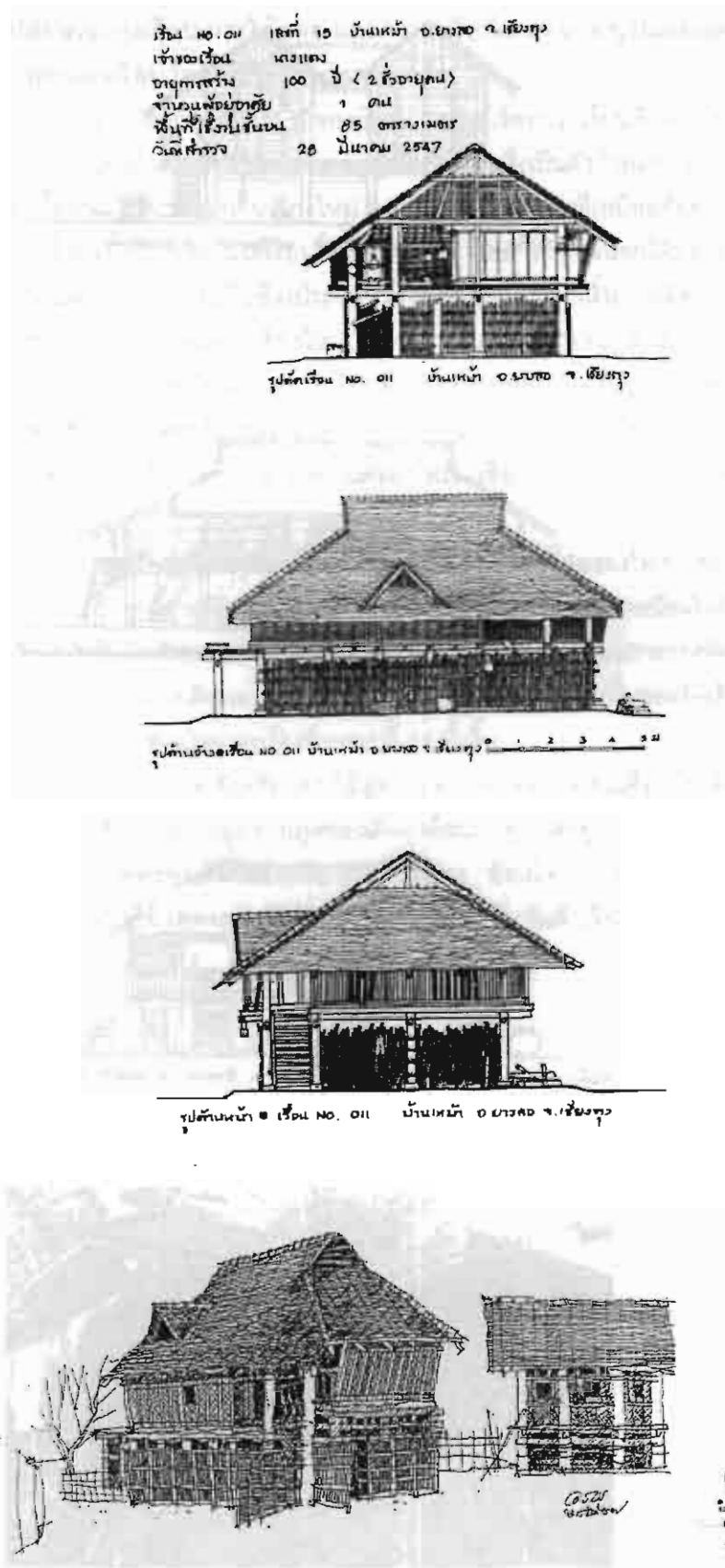
รูป 20 แสดงผังพื้น รูปตัด รูปด้าน และทัศนียภาพของเรือนนางแดง บ้านเลขที่ 15 บ้านหม้า อำเภอฝาง จังหวัดเชียงใหม่
