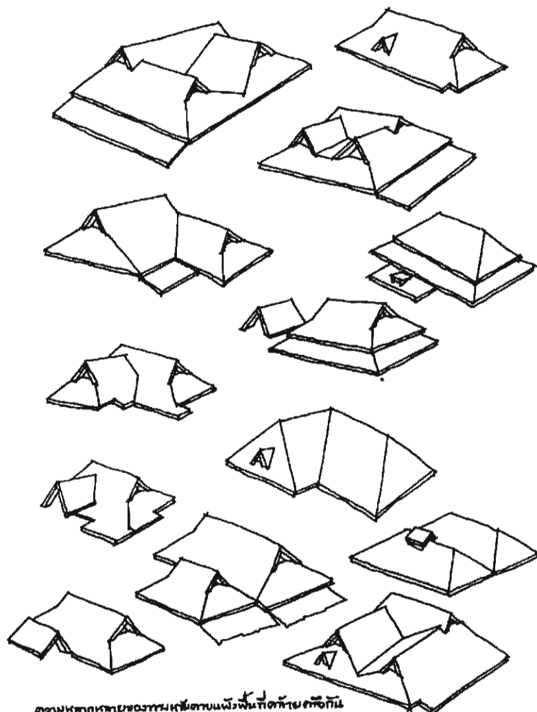
รูป 25 รูปทรงหลังคาเรือนไทเขินเชียงใหม่
