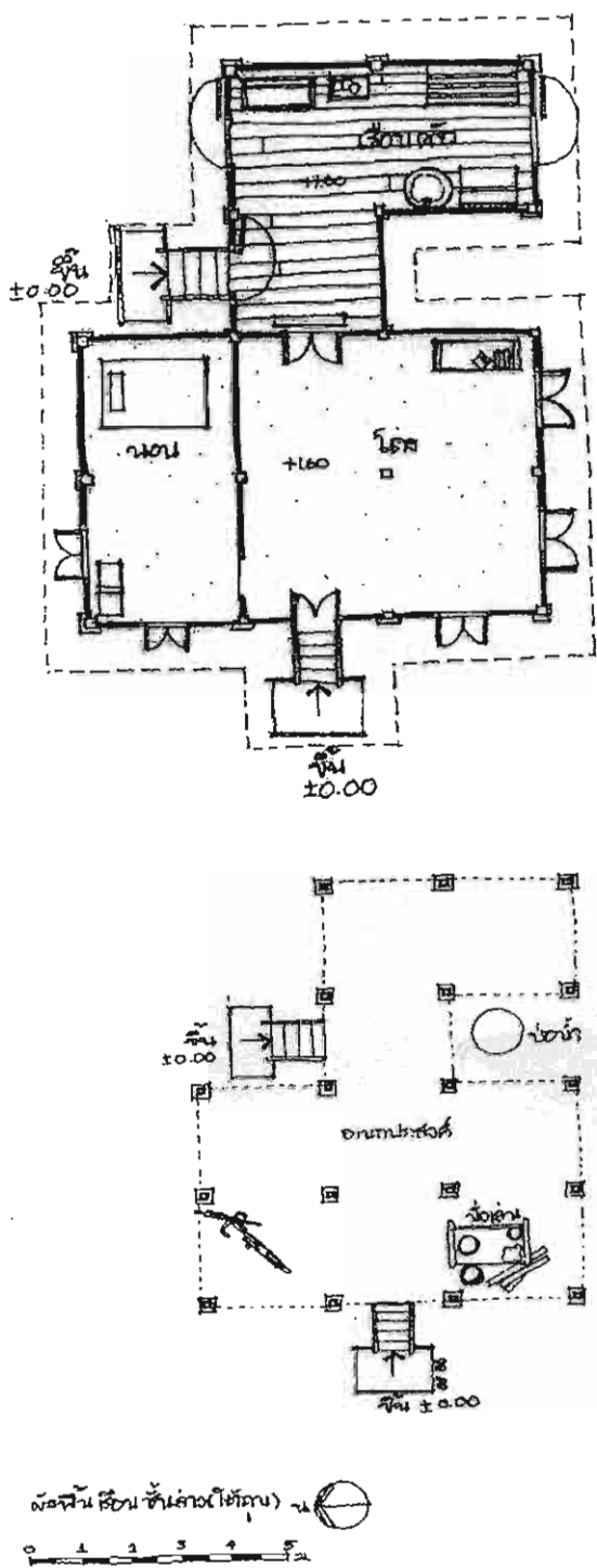
รูปที่ 3.65 ผังพื้นเรือนชั้นบนและใต้ดินเรือน
