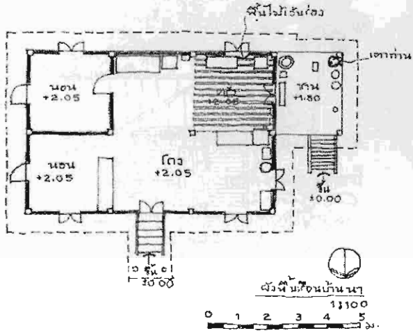
รูปที่ 3.11 ผังพื้นเรือน T1 นางชอคะ หลงทัน
