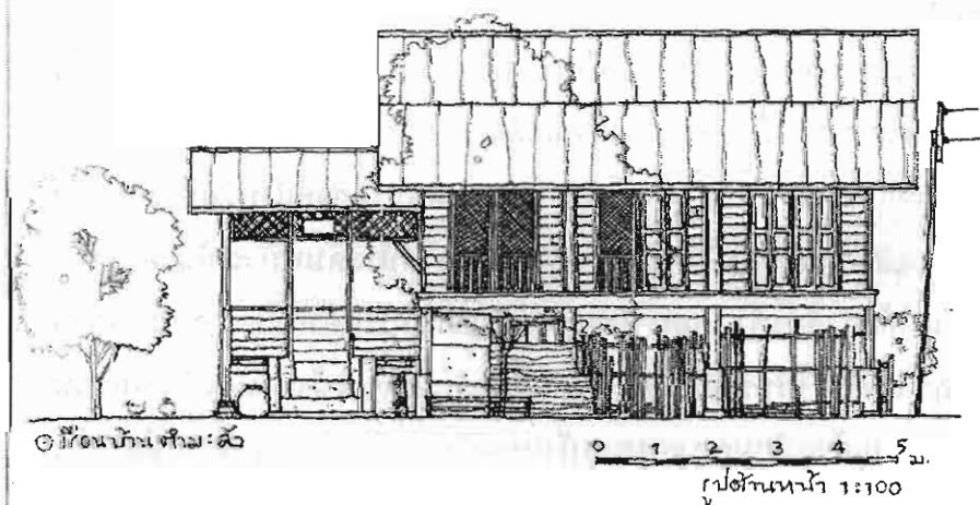
รูปที่ 3. 26 รูปด้านเรือนค้ำมะลัง
