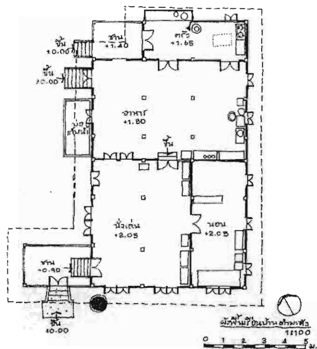
รูปที่ 3. 25 รูปผังพื้นเรือนค้ำมะลัง
