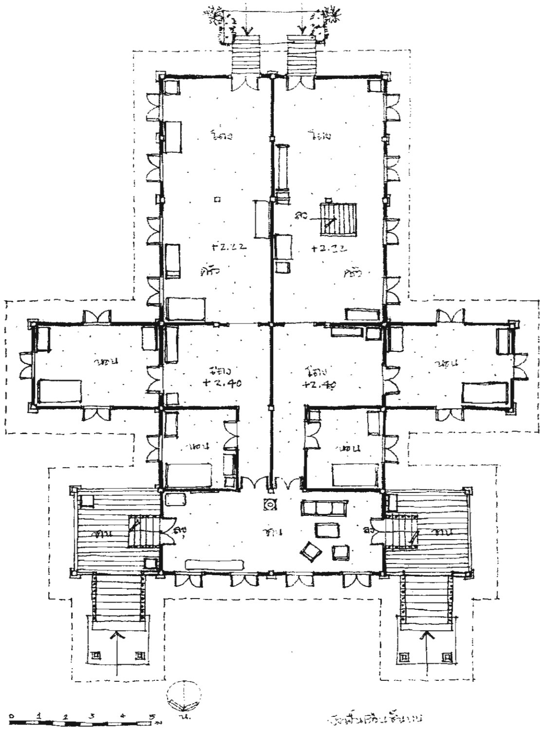
รูปที่ 3.94 ผังพื้นเรือน Abdul Jalil.
