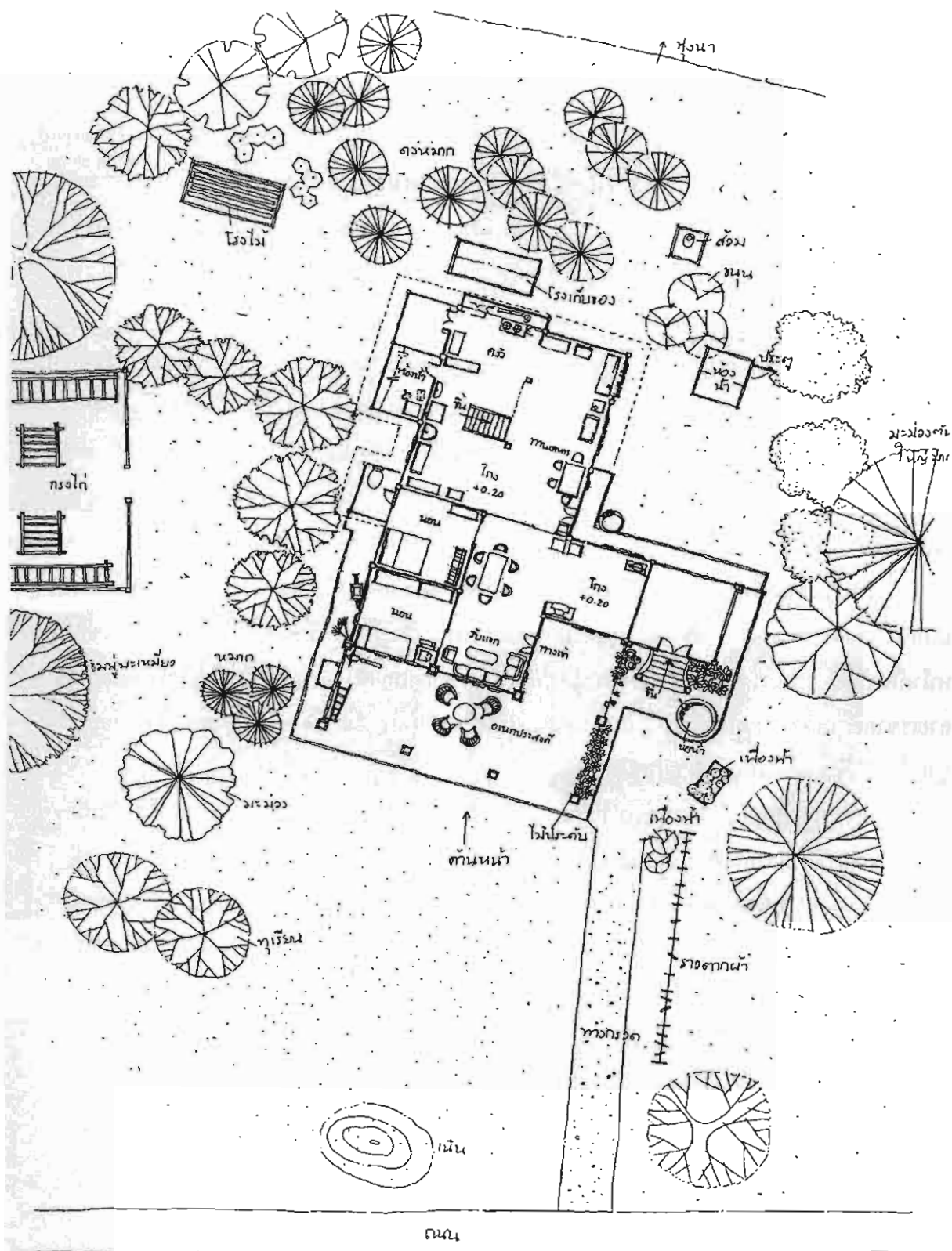
รูปที่ 3.102 ผังบริเวณเรือน Haji Abdulah Musa.
