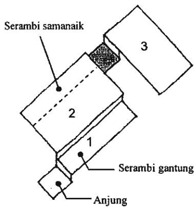
รูปที่ 4. 17 ภาพแสดงองค์ประกอบหลักของผังพื้นในเรือนพื้นถิ่นมุสลิม ที่พบในประเทศมาเลเซีย (ดัดแปลงจาก Yuan: 1987)
