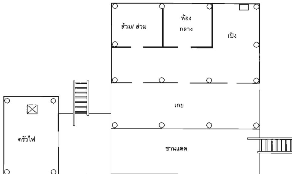
ภาพที่ 4-10 แสดงแบบแผนการกำหนดพื้นที่ของเรือนไท-ลาวในอีสาน
