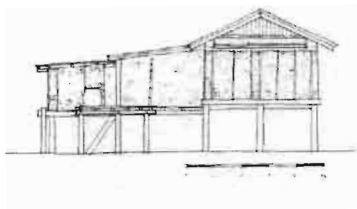
ภาพที่ 4-6 เรือนเกย ไทลาว จังหวัดกาฬสินธุ์และเรือนเขีย ไทย้อ จังหวัด นครพนม
