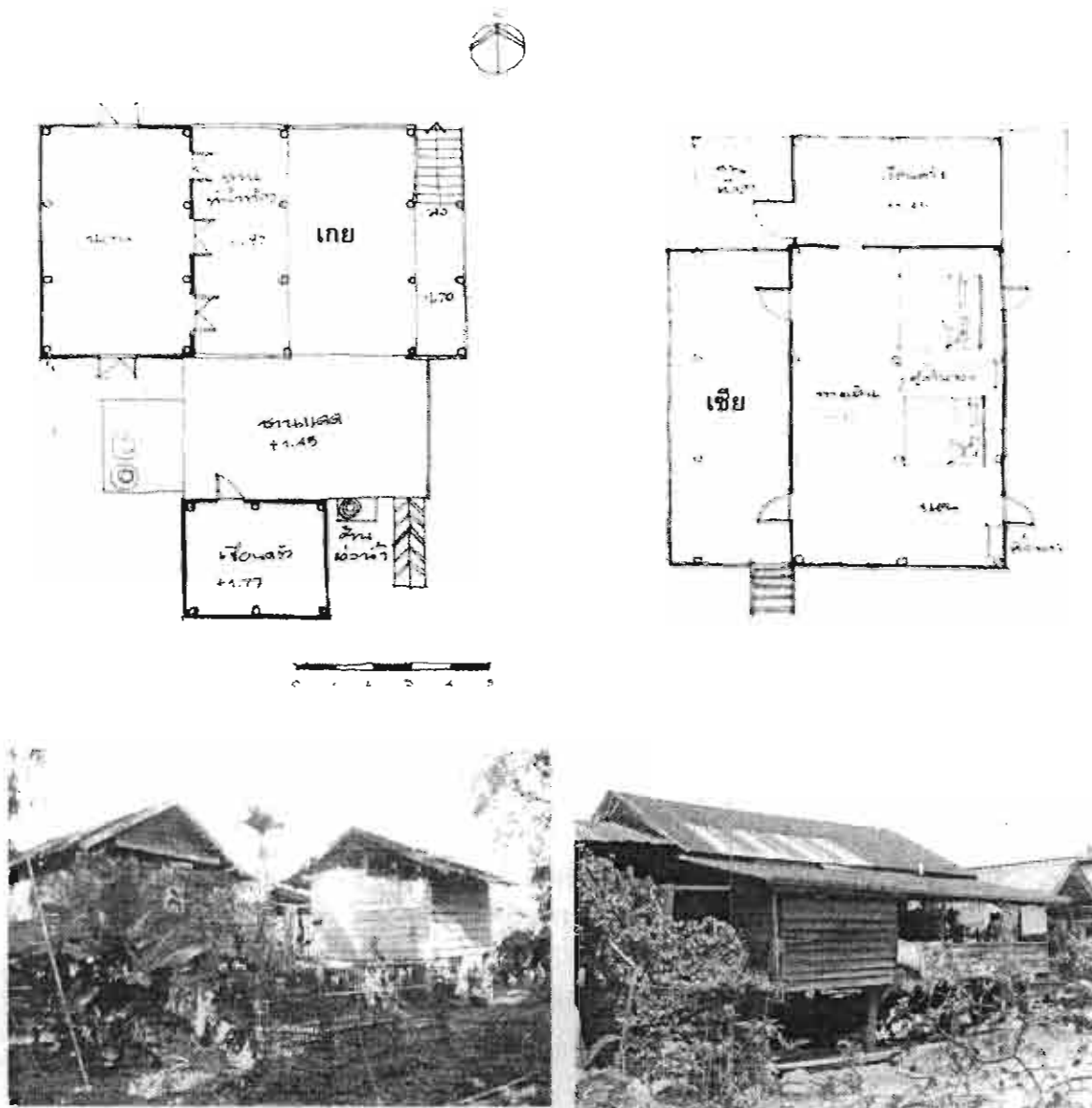
เรือนเกย ไทยย้อ บ้านจิว อำเภอกุดบาก จังหวัดสกลนคร
