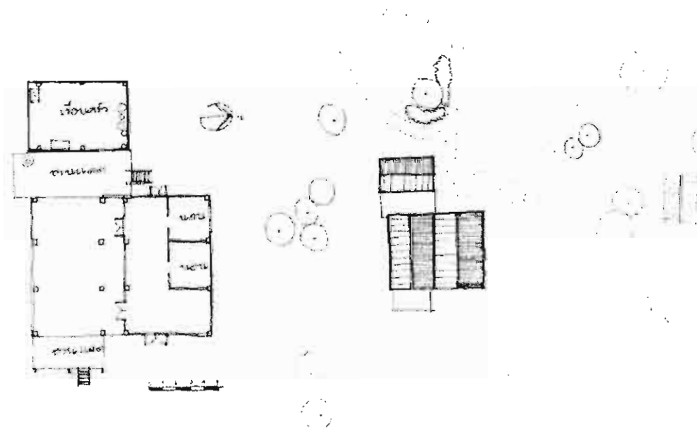
ภาพที่ 3-7 ผังพื้นเรือนและผังบริเวณ แสดงการวางทิศทางของเรือนผู้ไท เลขที่ 105 บ้านโนนยาง อำเภอนองสูง จังหวัดมุกดาหาร
