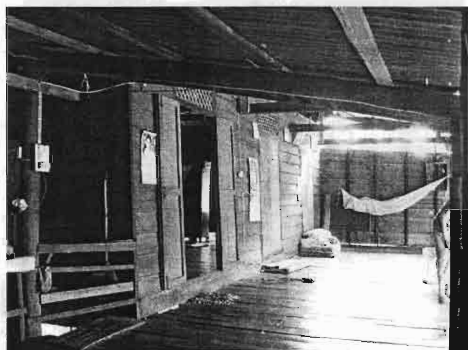
ภาพที่ 4-13 พื้นที่เกยหรือเชย ในเรือนไทยอีสาน บ้านโพธิ์ จังหวัดนครพนม
