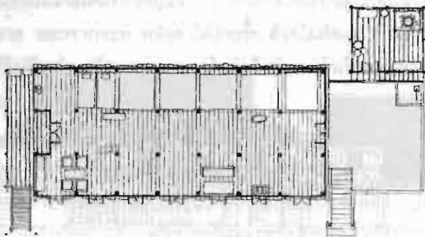
รูป 9.10 ก ผังพื้น
