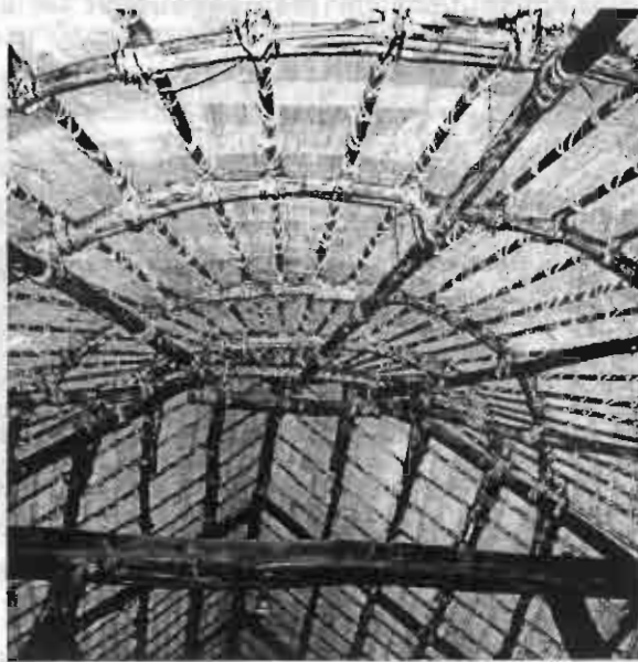
รูป 5.26 กวางตูปที่หลังคาด้านสกัด ใช้ไม้ไผ่รวก 5-6 ลำ มัดรวมกันดัดโค้ง
