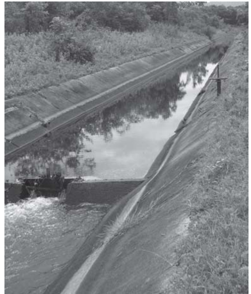
คลองส่งน้ำจากอ่างเก็บน้ำแม่ตูป
