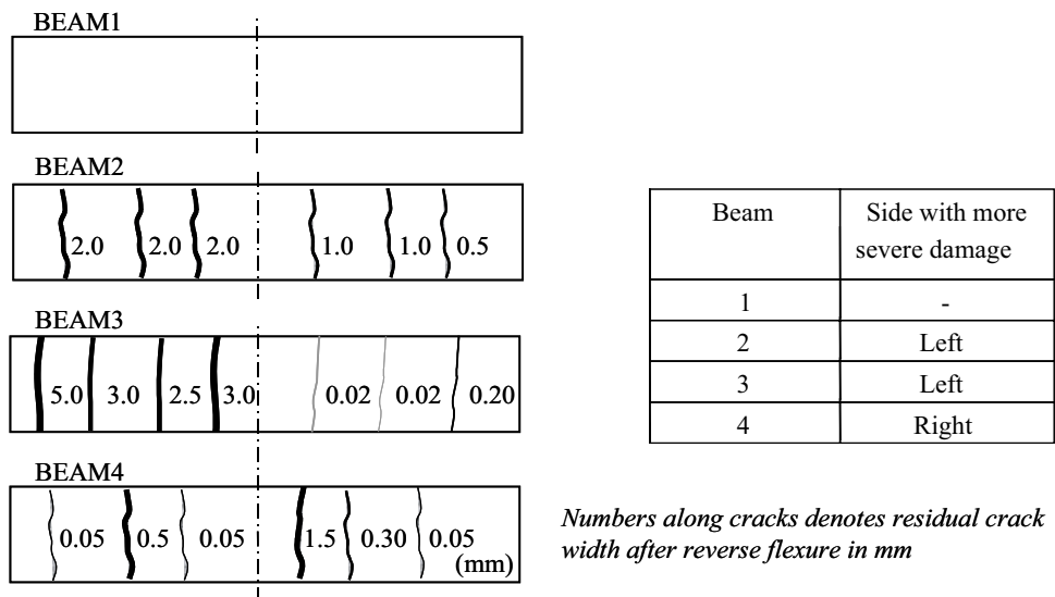
รูป 1.3 รอยร้าวที่เกิดขึ้นภายหลังการทดสอบการดัดกลับทิศ
