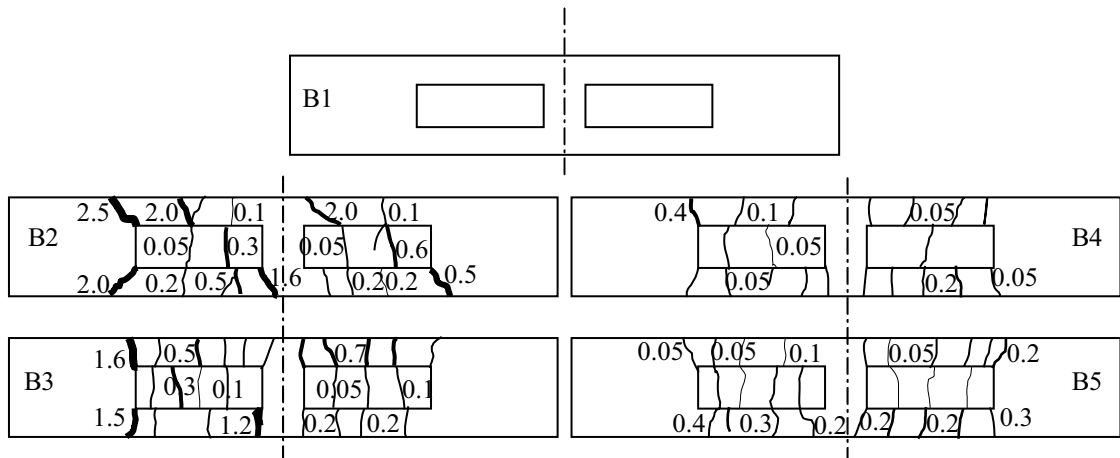
รูป 2.4 ความกว้างรอยร้าวที่ได้จากการทดสอบ 4 จุดสลับทิศ
