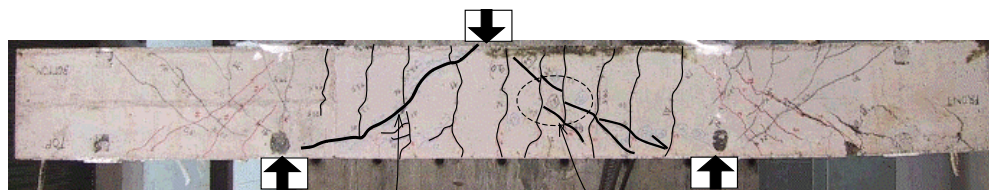
(c) น้ำหนักบรรทุกทุกชั้นที่ 3: การตัด 3 จุดรอบที่ 1
