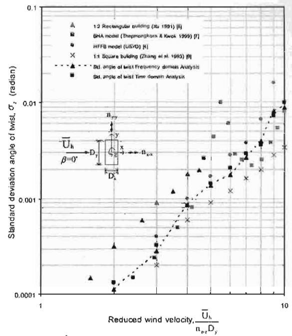
รูปที่ 5 การแอ่นตัวที่ระดับยอดของอาคาร CAARC ในแนวทิศ สำหรับความเร็วลมค่าต่างๆ เมื่อลมพัดปะทะตั้งฉากกับด้านยาวของอาคาร
