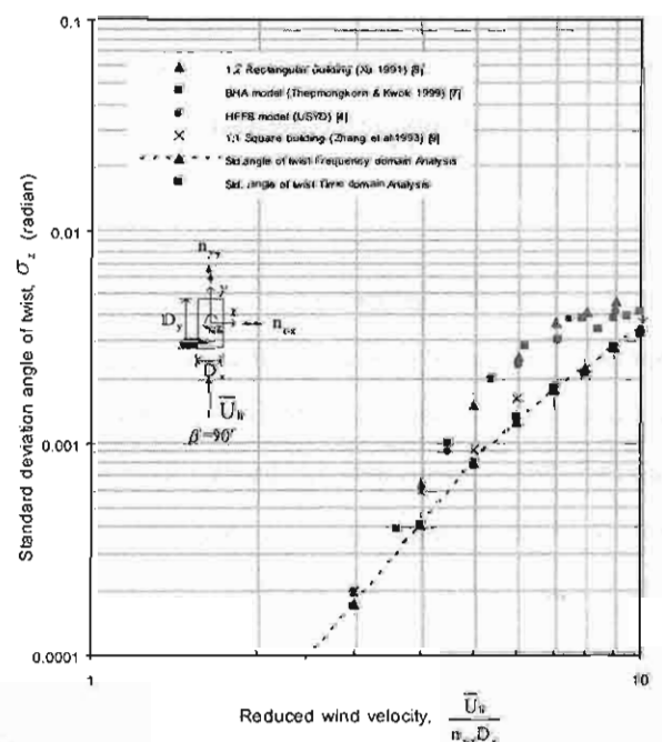
รูปที่ 6 การแอ่นตัวที่ระดับยอดของอาคาร CAARC ในแนวทิศ สำหรับความเร็วลมค่าต่างๆ เมื่อลมพัดปะทะตั้งฉากกับด้านกว้างของอาคาร
