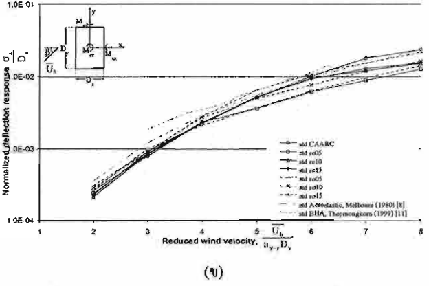
รูปที่ 5 ค่าเบี่ยงเบนมาตรฐานของการแอ่นตัวของอาคารที่ระดับยอดอาคารในทิศทางตั้งฉากกับกระแสลม (ก) \beta = 0 องศา (ข) \beta = 90 องศา
