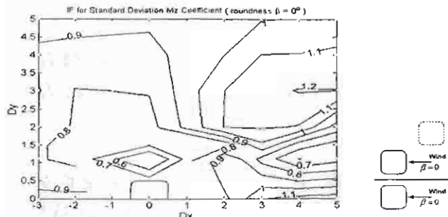
(ง) หน้าตัดสี่เหลี่ยมจัตุรัสผืนดินมน
