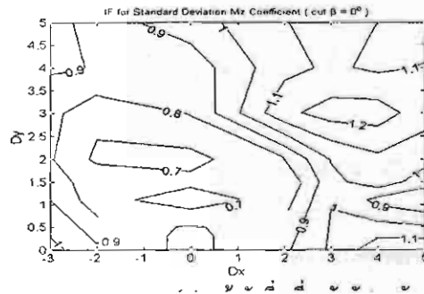
(ข) หน้าตัดสี่เหลี่ยมจัตุรัสแนว
