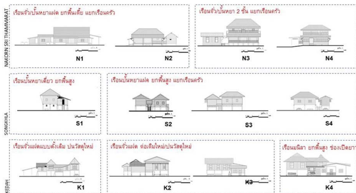
ภาพที่ 4.7 การเปรียบเทียบเรือน 1) ชุมชนแหลมและเขาพังไกร (ในพื้นที่ต่อเนื่องกัน) อ.หัวไทร จ. นครศรีธรรมราช 2) ชุมชนคูเต่า อ.หาดใหญ่ และอ.บางกล่ำ (ในพื้นที่ต่อเนื่องกัน) จ.สงขลา และ3) ชุมชนปลายระไม ต.ทุ่งควาย อ.เป็นดั่ง รัฐเกดะห์ ในมาเลเซีย
