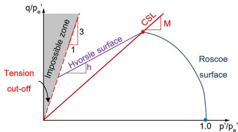
รูปที่ 2.24 พื้นผิวครากของดินเหนียว (yield surface of clays) (สุเชษฐ์ 2553)
