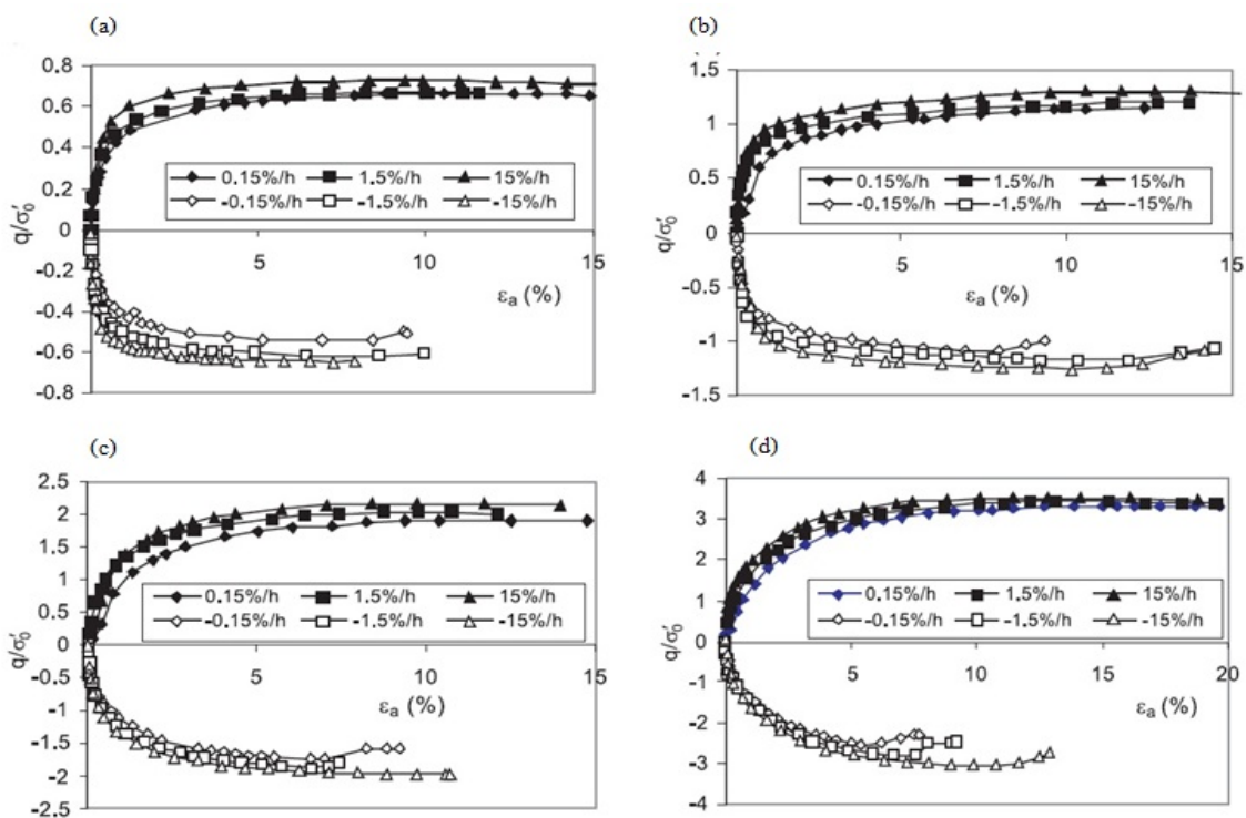
รูปที่ 2.39 ความสัมพันธ์ระหว่างการค่าความเค้นเบี่ยงเบนประสิทธิผล กับความเครียดแนวแกนของ Zhu และ Yin (1999) (a) OCR= 1 (b) OCR= 2 (c) OCR= 4 (d) OCR= 8
