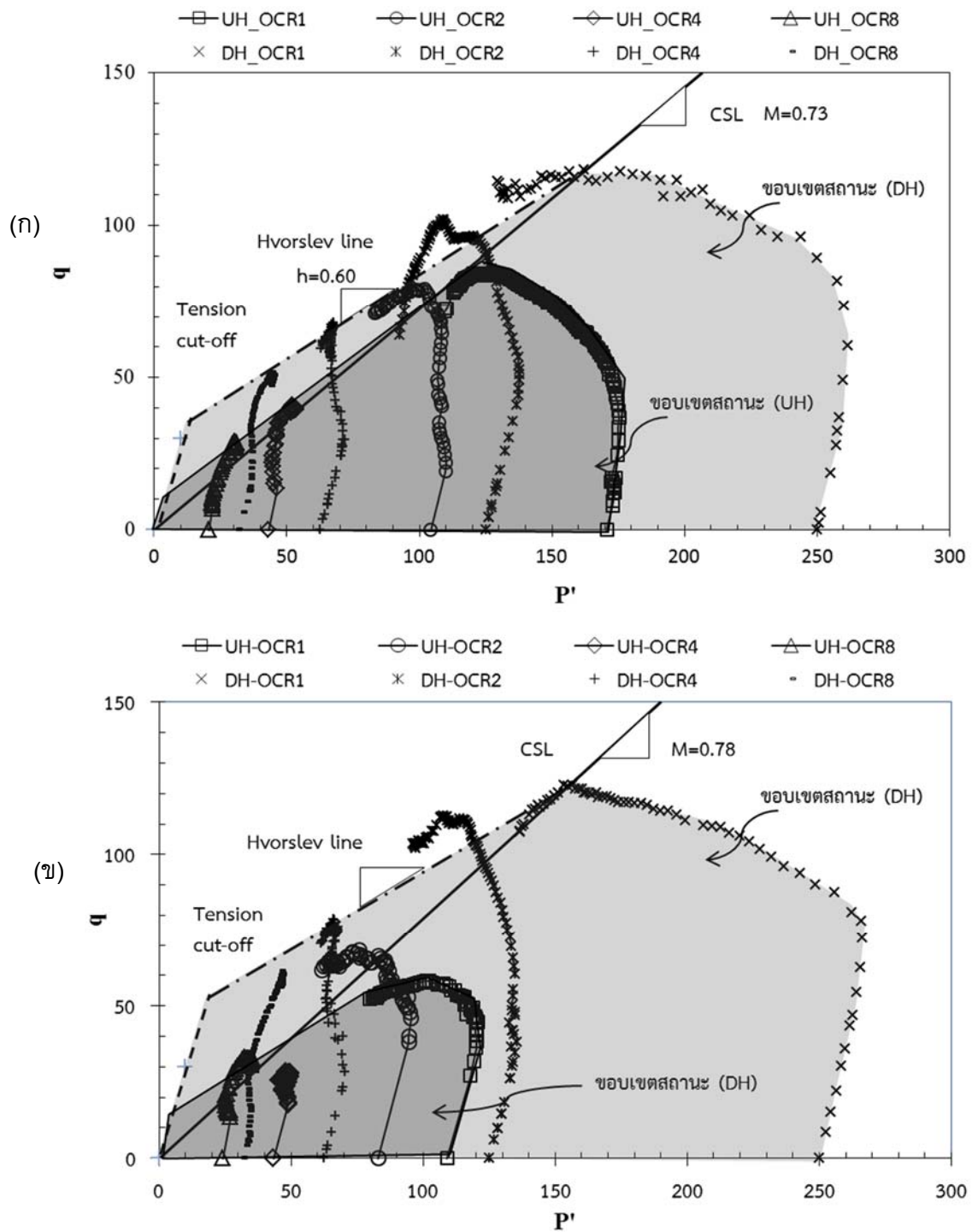
รูปที่ 4.51 เส้นทางความเค้นที่ค่าการอัดแน่นเกินตัวแตกต่างกันอัตราความเครียด 0.075% มม.ต่อนาที (ก) อุนหนุมมี 45 องศาเซลเซียส (ข) อุนหนุมมี 60 องศาเซลเซียส
