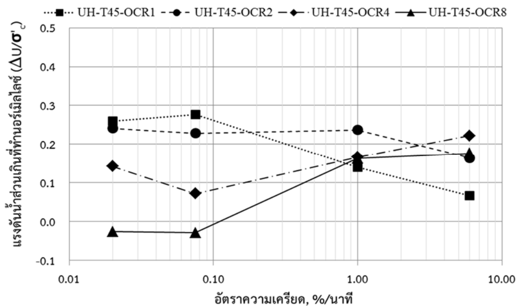
รูปที่ 4.28 ความสัมพันธ์ระหว่างแรงดันน้ำส่วนเกินที่ทำการนอร์เมลไลซ์ กับอัตราความเครียดที่อุณหภูมิ 45 องศาเซลเซียส
