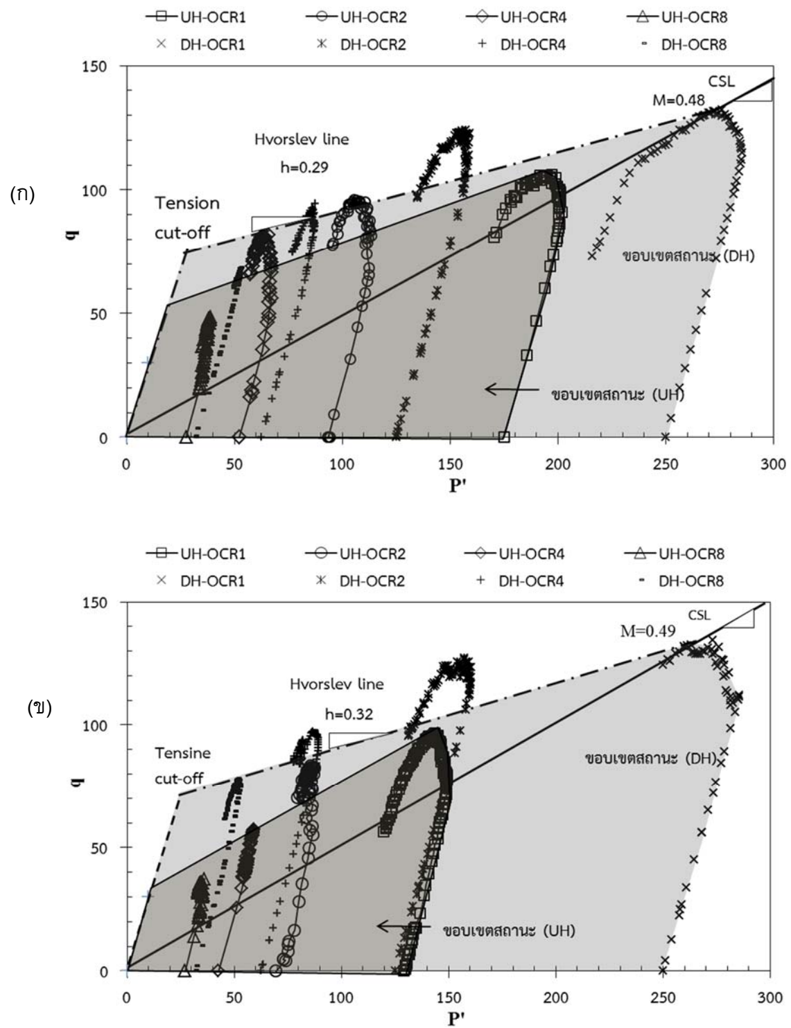
รูปที่ 4.53 เส้นทางความเค้นที่ค่าการอัดแน่นเกินตัวแตกต่างกัน อัตราความเครียด 6.0% มม.ต่อนาที (ก) อุณหภูมิ 45 องศาเซลเซียส (ข) อุณหภูมิ 60 องศาเซลเซียส
