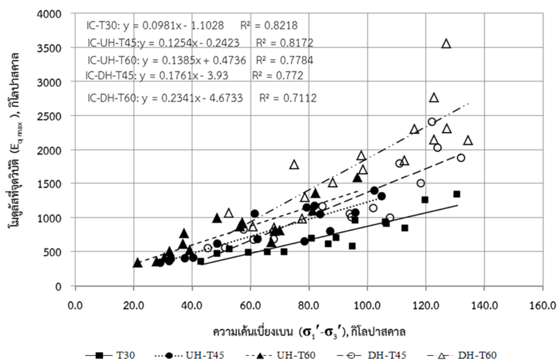
รูปที่ 4.38 กราฟความสัมพันธ์ระหว่างค่าโมดูลัสยืดหยุ่นกับค่าความเค้นเบี่ยงเบนสูงสุดของดินเหนียวปากพั้งทดสอบที่อุณหภูมิ 30 45 และ 60 องศาเซลเซียส
