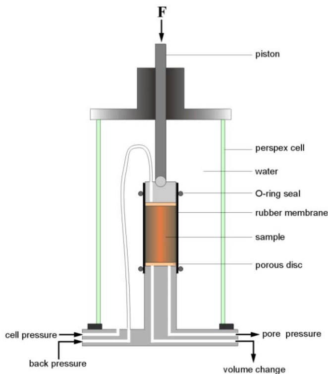
รูปที่ 2.17 เครื่องมือทดสอบแรงอัดสามแกน ( https://www.gdsinstruments.com )
