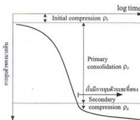
(ข) การยุบตัวของมวลดินกับล็อกของเวลา (Soil compression vs. log time)
